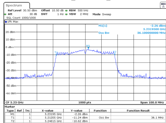
802.11ac40_5230MHz_Chain 1
