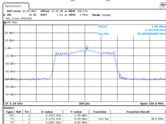
802.11ac40_5190MHz_Chain 2
