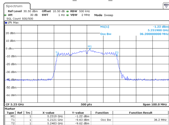
802.11ac40_5230MHz_Chain 2
