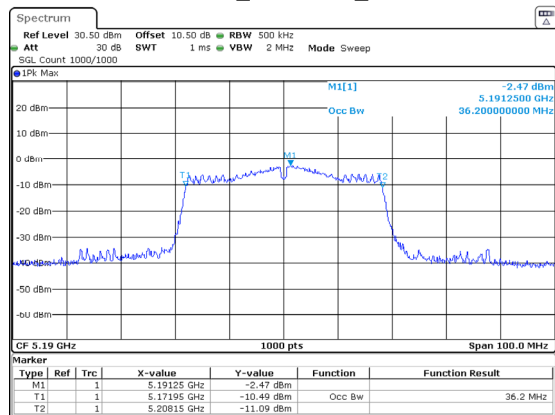
802.11ac40_5190MHz_Chain 1
