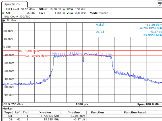
802.11ac40_5755MHz_Chain 1
