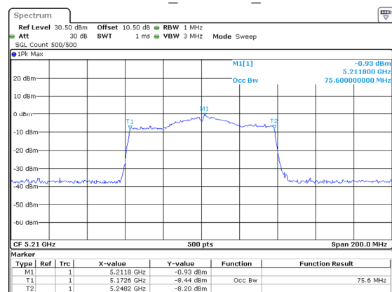
802.11ac80_5210MHz_Chain 2
