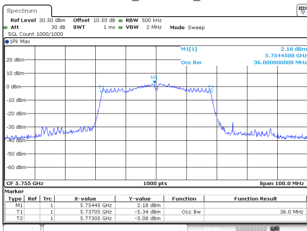
802.11ac40_5755MHz_Chain 1
