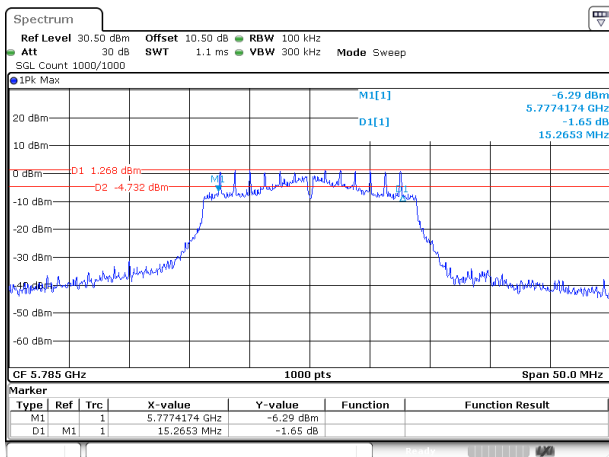
802.11ac20_5785MHz_Chain 1
