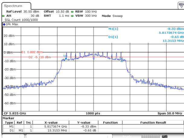
802.11ac20_5825MHz_Chain 0
