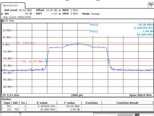
802.11ac80_5210MHz_Chain 1
