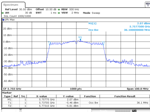
802.11ac40_5755MHz_Chain 0
