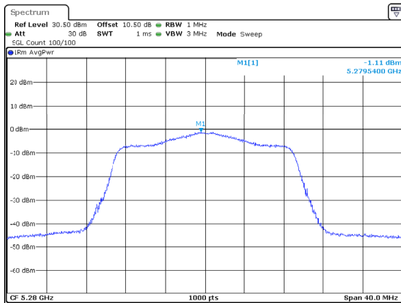
802.11ac20_5280MHz_Chain 2
