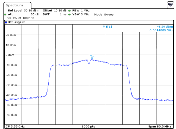
802.11ac40_5550MHz_Chain 2
