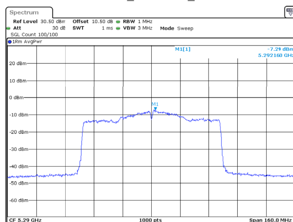
802.11ac80_5290MHz_Chain 2
