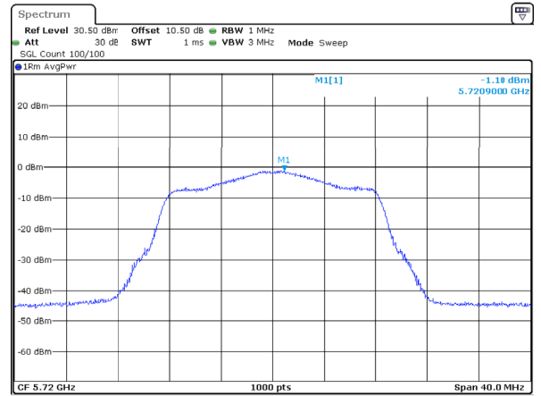
802.11a_5720MHz_Chain 2
