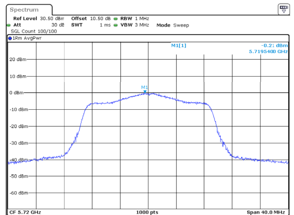
802.11ac20_5720MHz_Chain 1
