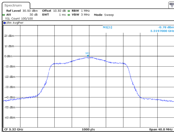
802.11ac20_5320MHz_Chain 1
