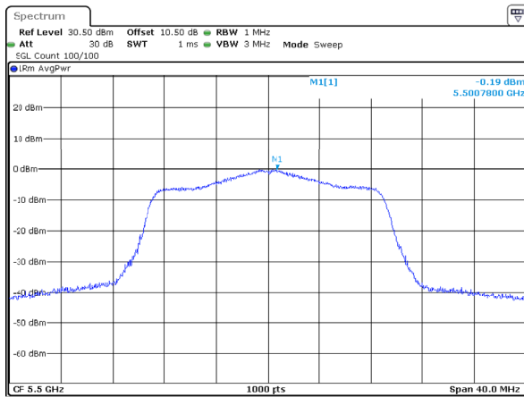
802.11ac20_5500MHz_Chain 1
