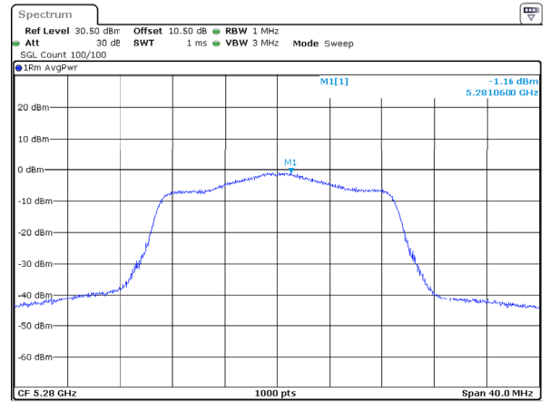
802.11ac20_5280MHz_Chain 1
