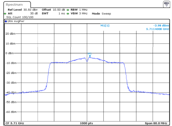
802.11ac40_5710MHz_Chain 1
