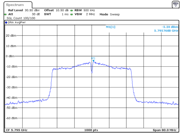
802.11ac40_5795MHz_Chain 2
