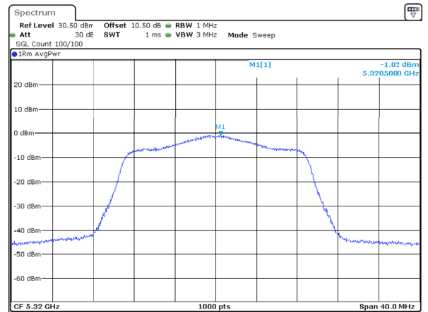
802.11ac20_5320MHz_Chain 2
