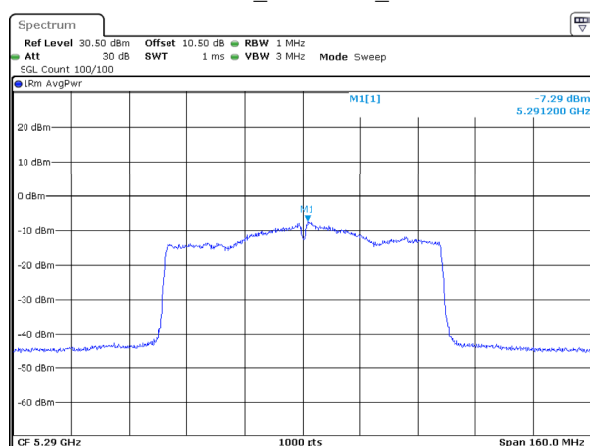
802.11ac80_5290MHz_Chain 1
