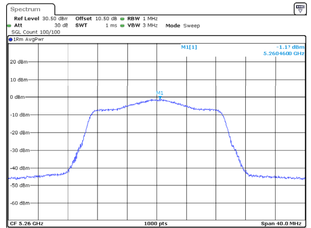
802.11ac20_5260MHz_Chain 2
