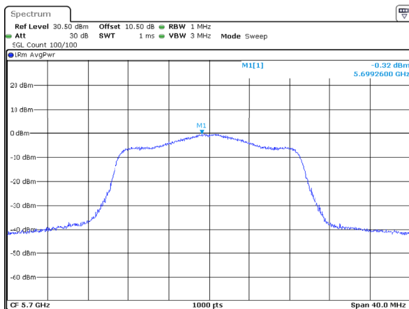
802.11ac20_5700MHz_Chain 1
