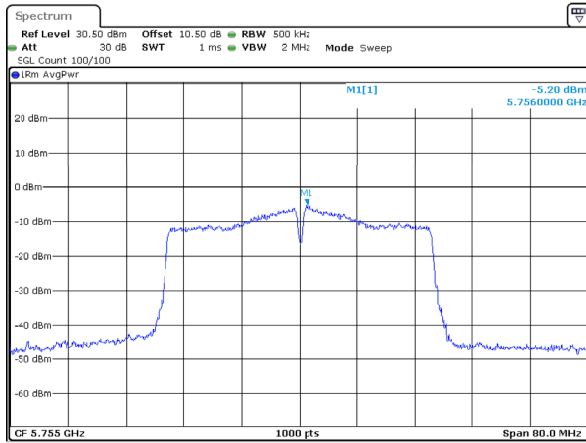
802.11ac40_5755MHz_Chain 2
