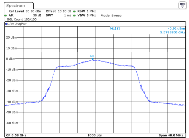
802.11ac20_5580MHz_Chain 1
