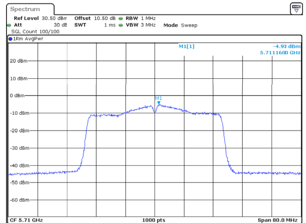
802.11ac40_5710MHz_Chain 2
