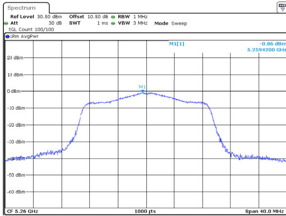
802.11ac20_5260MHz_Chain 1
