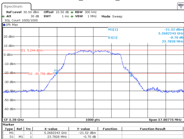
802.11ac20_5280MHz_Chain 1
