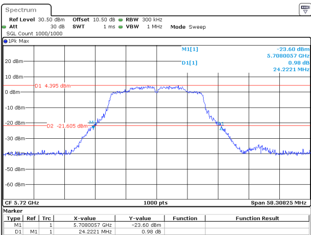
802.11ac20_5720MHz_Chain 1
