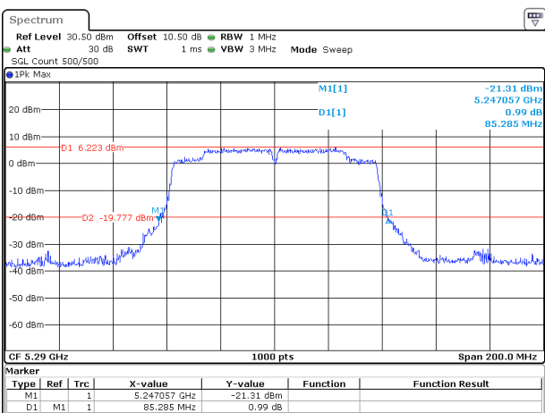
802.11ac80_5290MHz_Chain 0
