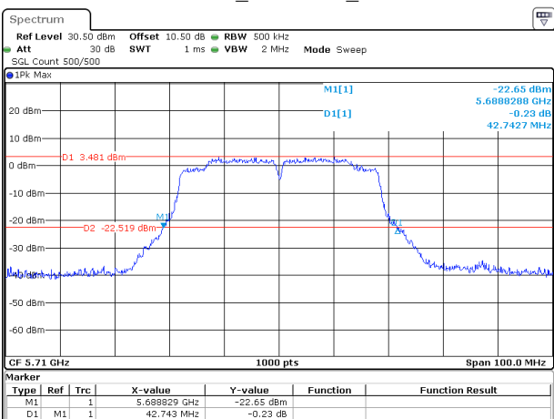
802.11ac40_5710MHz_Chain 0
