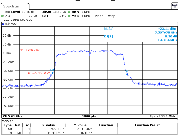
802.11ac80_5610MHz_Chain 0
