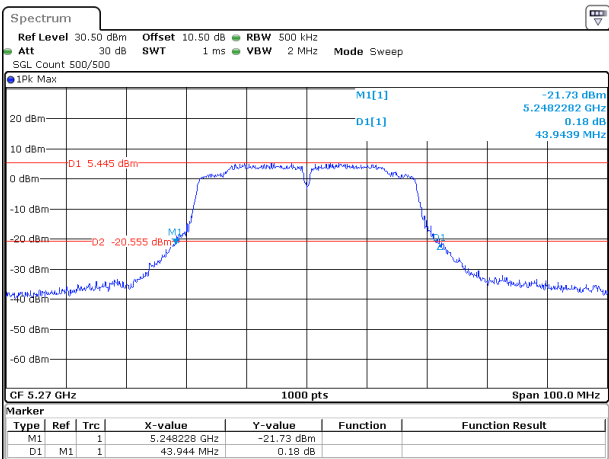
802.11ac40_5270MHz_Chain 1
