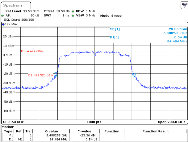
802.11ac80_5530MHz_Chain 1
