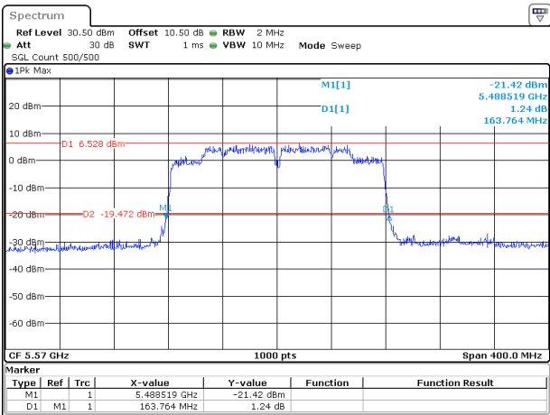
802.11ac160_5570MHz_Chain 1
