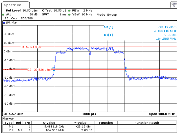
802.11ac160_5570MHz_Chain 0
