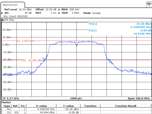
802.11ac40_5270MHz_Chain 0
