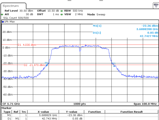
802.11ac40_5710MHz_Chain 1
