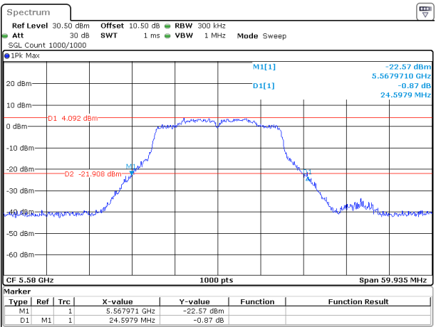
802.11ac20_5580MHz_Chain 1
