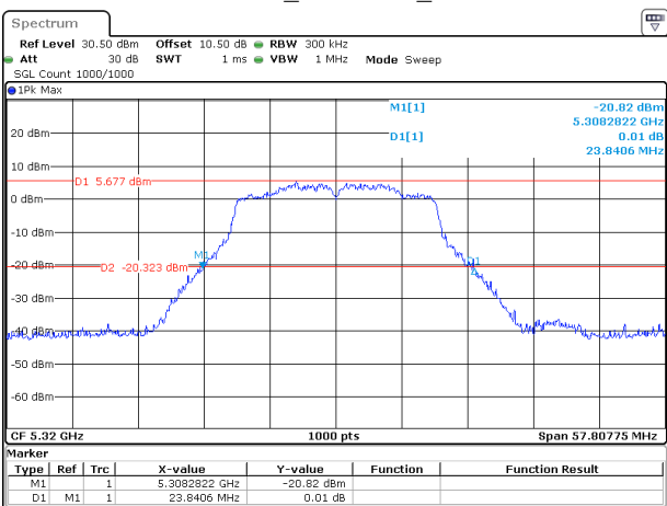
802.11ac20_5320MHz_Chain 1
