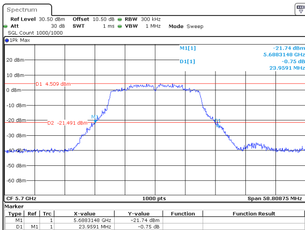
802.11ac20_5700MHz_Chain 1
