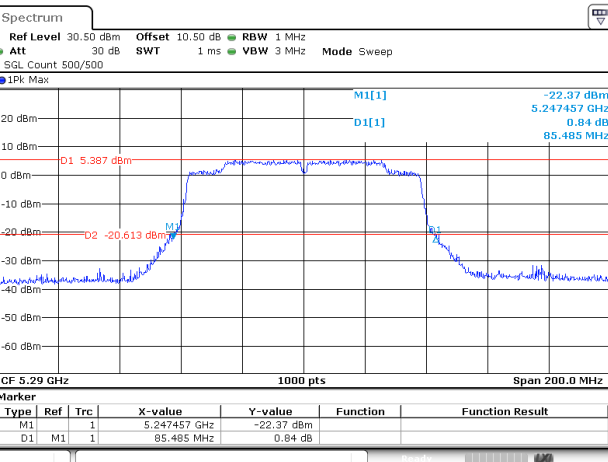
802.11ac80_5290MHz_Chain 1
