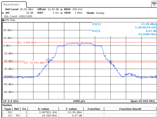
802.11ac20_5500MHz_Chain 1
