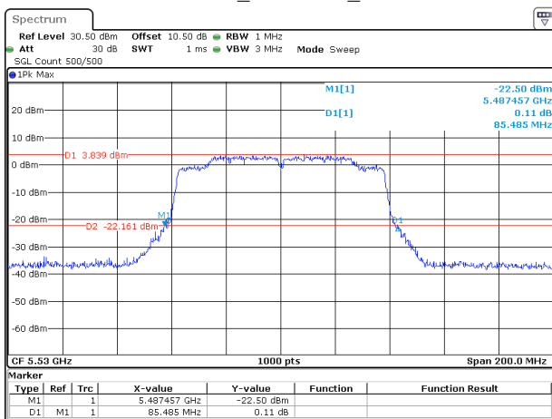
802.11ac80_5530MHz_Chain 0
