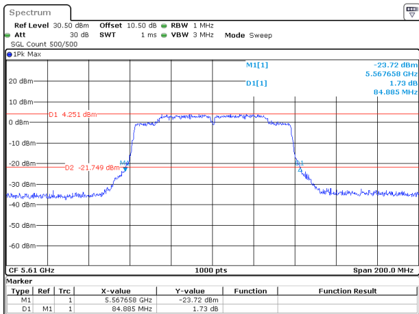
802.11ac80_5610MHz_Chain 1
