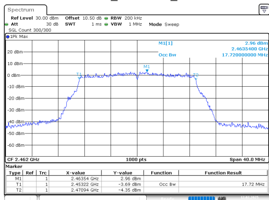
802.11n20_2462MHz_Chain 0
