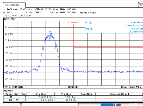
802.11b_2462MHz_Chain 0
