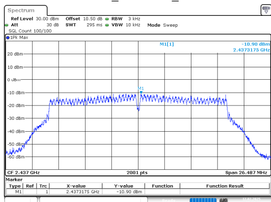
802.11n20_2437MHz_Chain 1
