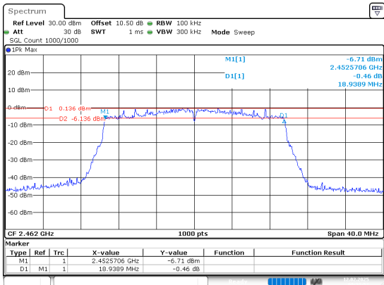
802.11ax20_2462MHz_Chain 1
