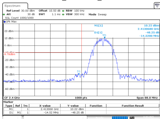
802.11b_2412MHz_Chain 1
