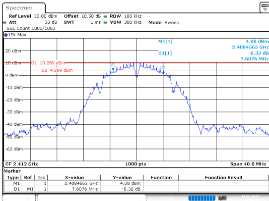
802.11b_2412MHz_Chain 1
