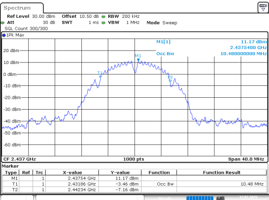
802.11b_2437MHz_Chain 1
