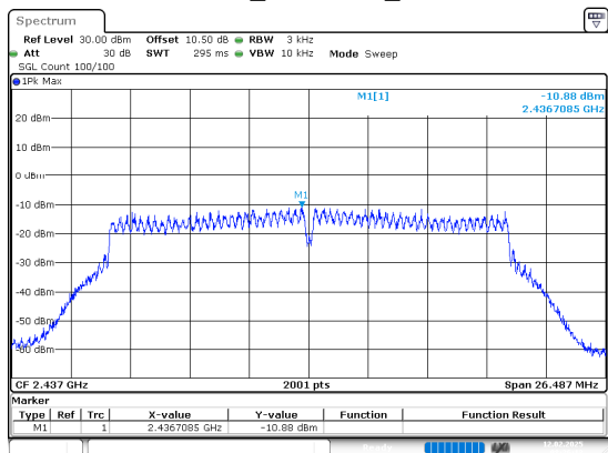
802.11n20_2437MHz_Chain 0
