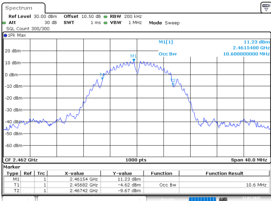
802.11b_2462MHz_Chain 1
