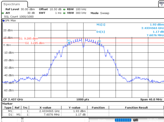
802.11b_2437MHz_Chain 0
