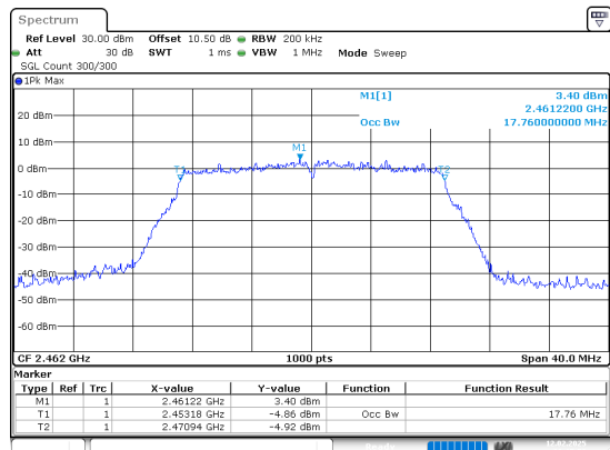
802.11n20_2462MHz_Chain 1
