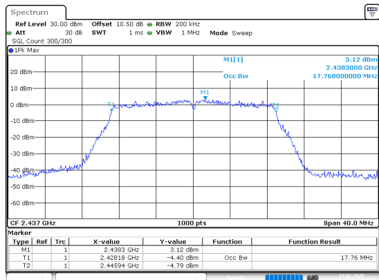
802.11n20_2437MHz_Chain 1
