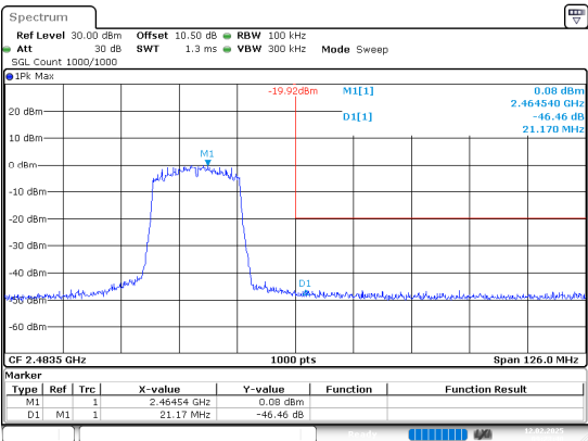
802.11ax20_2462MHz_Chain 1
