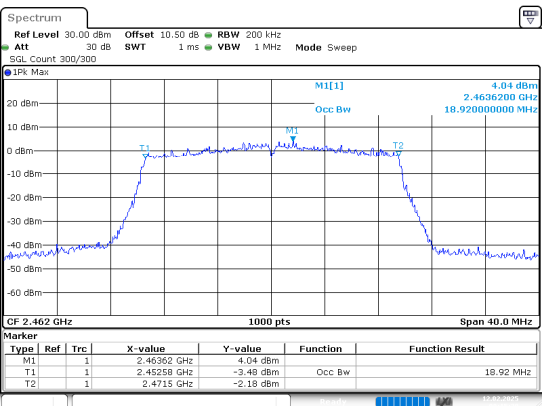
802.11ax20_2462MHz_Chain 0
