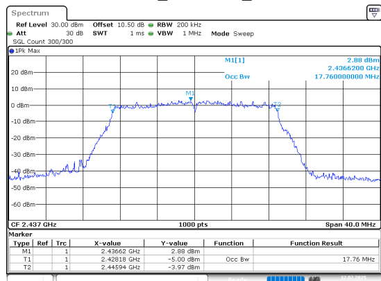
802.11n20_2437MHz_Chain 0
