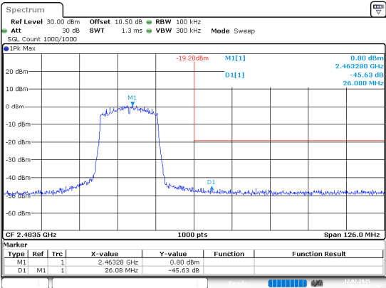
802.11ax20_2462MHz_Chain 0
