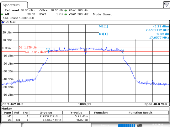
802.11n20_2462MHz_Chain 1
