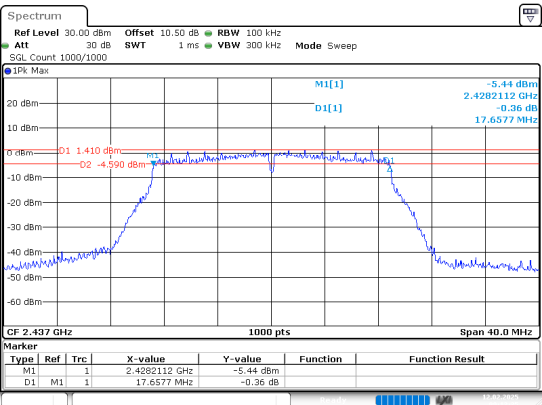
802.11n20_2437MHz_Chain 1
