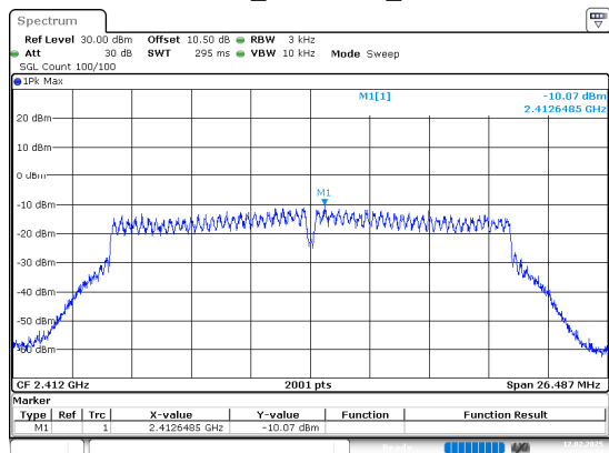
802.11n20_2412MHz_Chain 0
