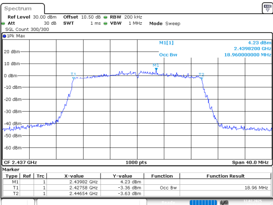
802.11ax20_2437MHz_Chain 0
