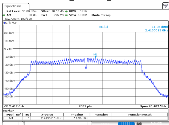
802.11n20_2412MHz_Chain 1
