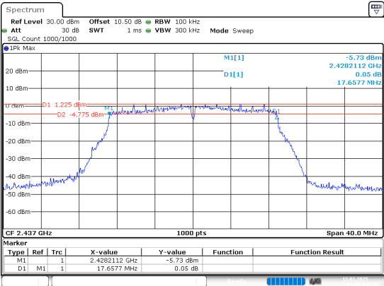
802.11n20_2437MHz_Chain 0
