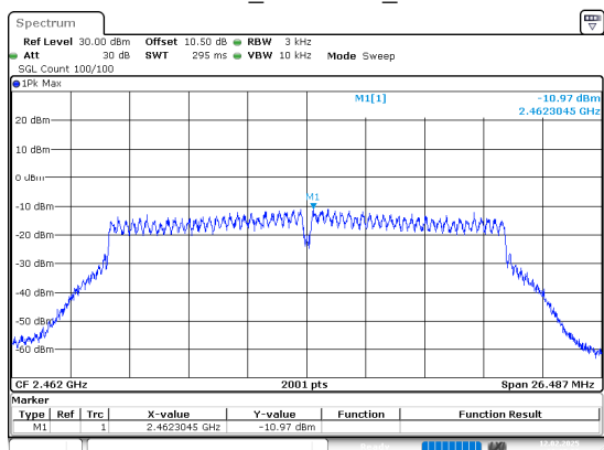
802.11n20_2462MHz_Chain 1
