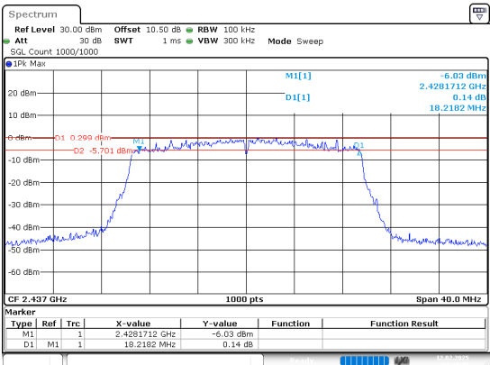
802.11ax20_2437MHz_Chain 1
