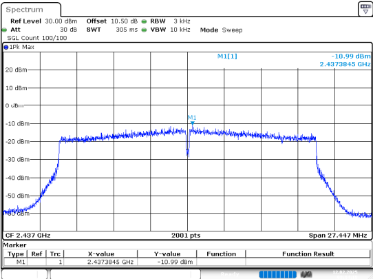
802.11ax20_2437MHz_Chain 0
