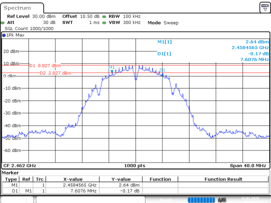
802.11b_2462MHz_Chain 0
