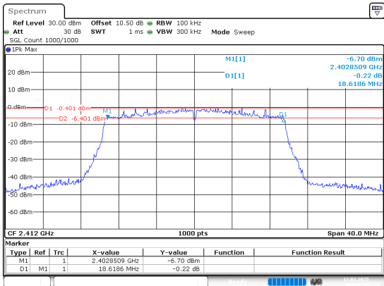
802.11ax20_2412MHz_Chain 1
