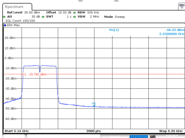
802.11n40_5190MHz_Chain 0
