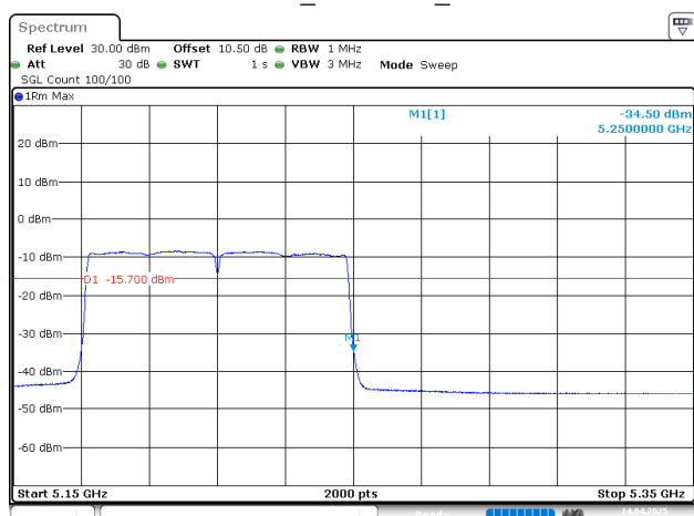
802.11ac80_5210MHz_Chain 0
