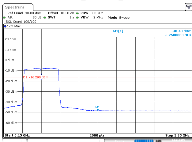
802.11n40_5190MHz_Chain 1
