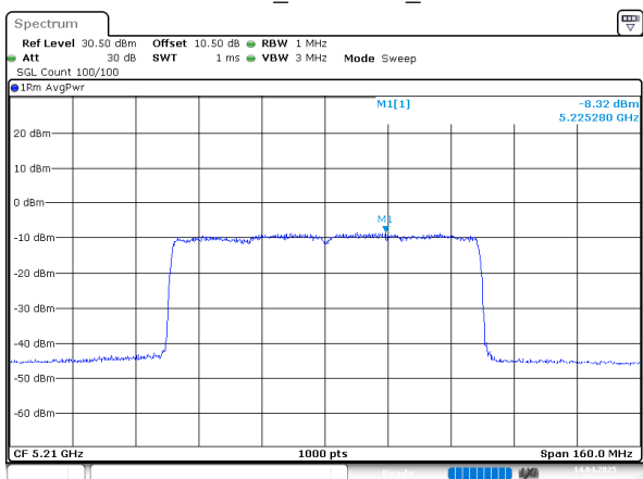
802.11ax80_5210MHz_Chain 1
