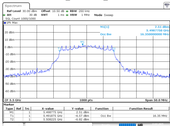
802.11a_5500MHz_Chain 1
