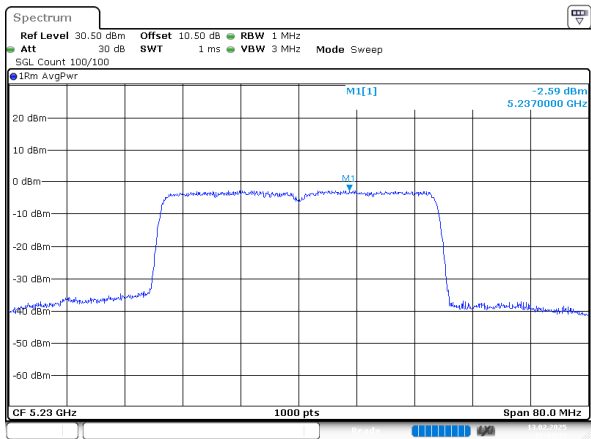
802.11ax40_5230MHz_Chain 0
