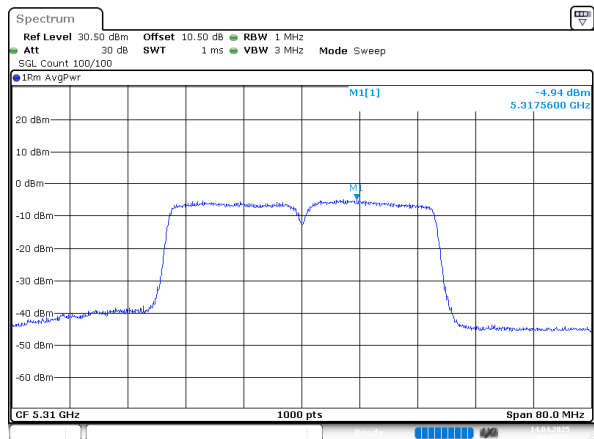
802.11n40_5310MHz_Chain 1
