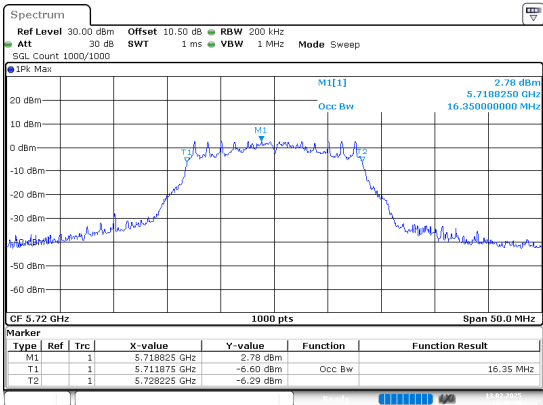
802.11a_5720MHz_Chain 1
