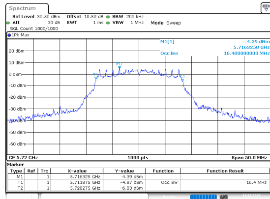
802.11a_5720MHz_Chain 0
