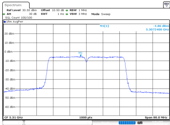
802.11n40_5310MHz_Chain 0
