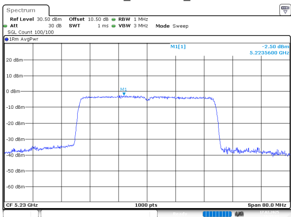
802.11ax40_5230MHz_Chain 1
