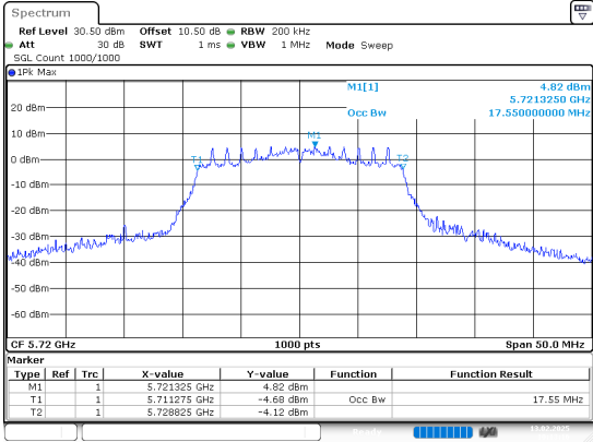
802.11n20_5720MHz_Chain 0
