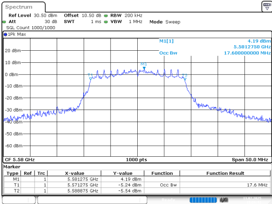
802.11n20_5580MHz_Chain 0
