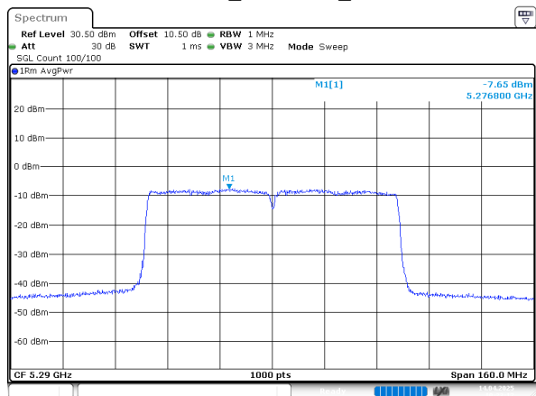
802.11ac80_5290MHz_Chain 1
