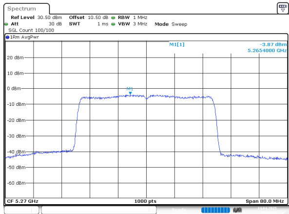
802.11ax40_5270MHz_Chain 0
