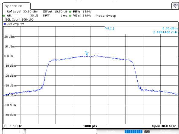
802.11ax20_5500MHz_Chain 1
