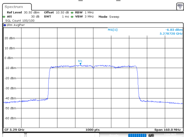
802.11ax80_5290MHz_Chain 0
