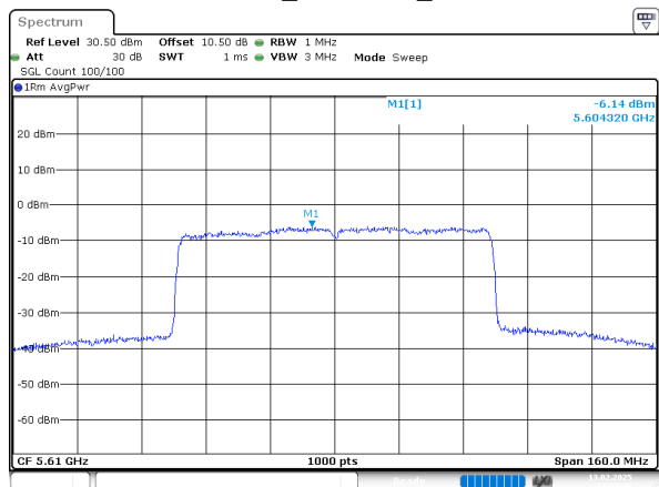
802.11ax80_5610MHz_Chain 0
