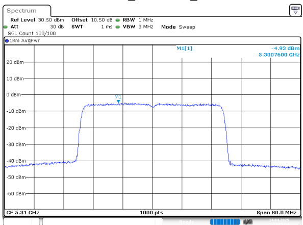
802.11ax40_5310MHz_Chain 1
