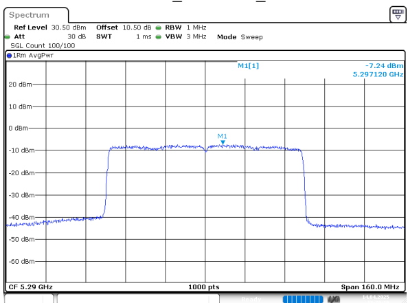
802.11ax80_5290MHz_Chain 1
