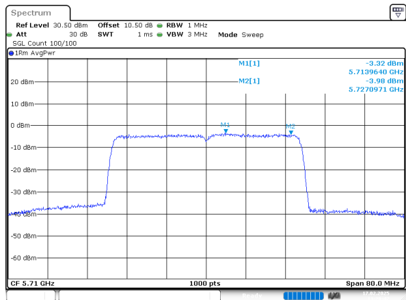
802.11ax40_5710MHz_Chain 1
