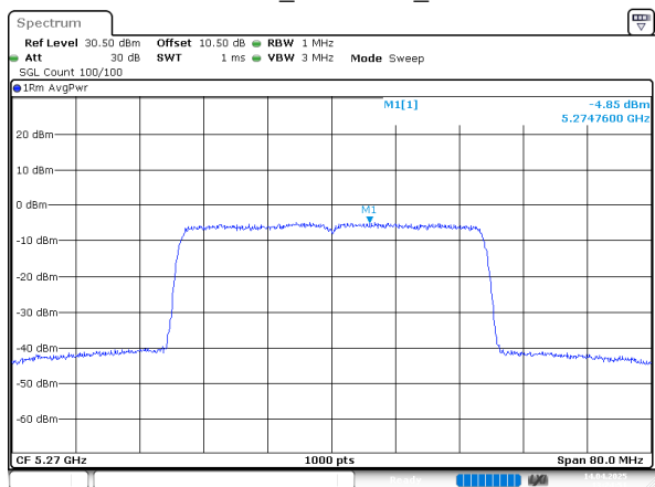
802.11ax40_5270MHz_Chain 1
