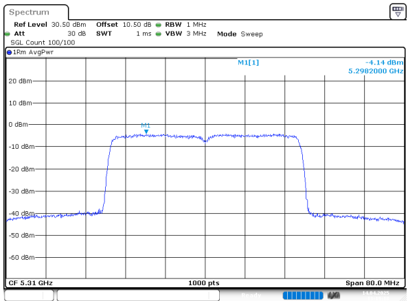
802.11ax40_5310MHz_Chain 0
