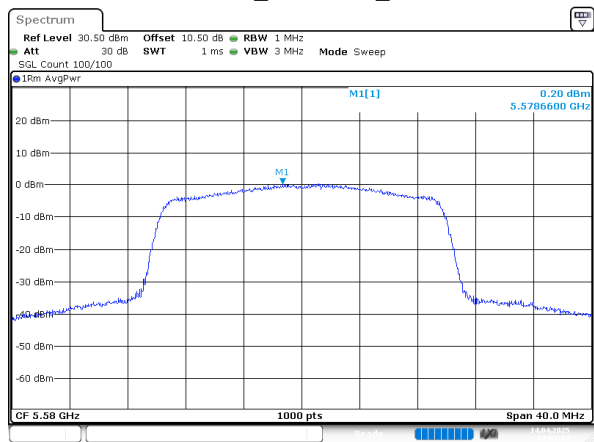
802.11ax20_5580MHz_Chain 1
