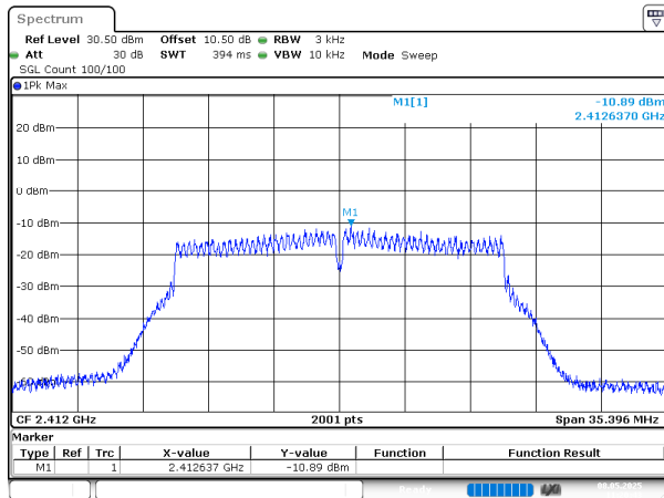
802.11n20_2412MHz_Chain 0
