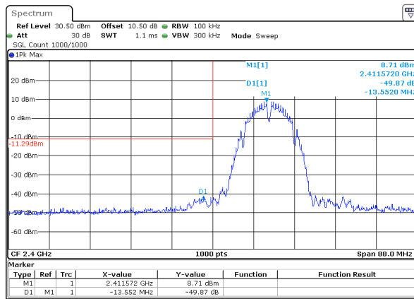
802.11b_2412MHz_Chain 1
