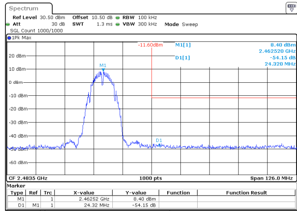
802.11b_2462MHz_Chain 0
