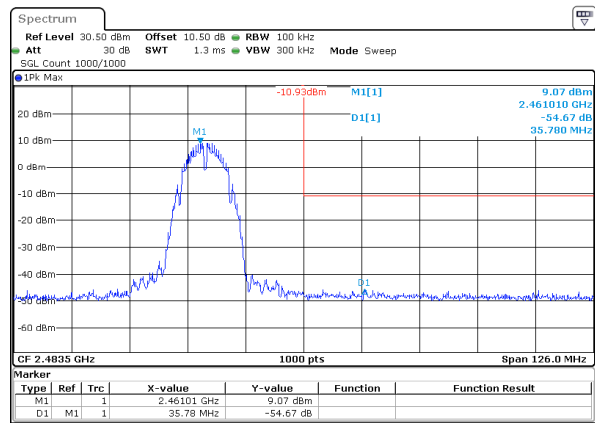
802.11b_2462MHz_Chain 1
