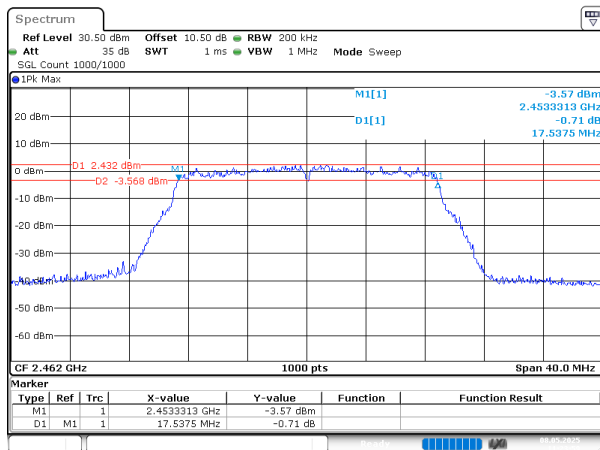
802.11n20_2462MHz_Chain 0
