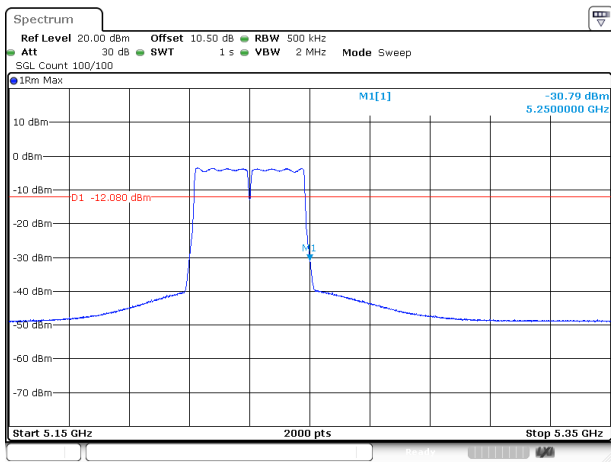
802.11ac40_5230MHz
