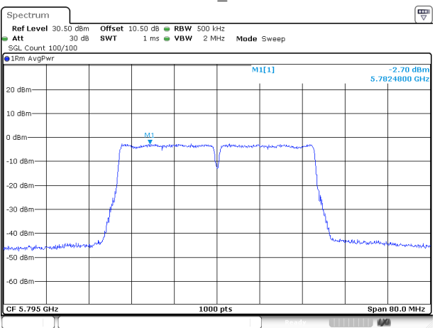
802.11ac40_5795MHz
