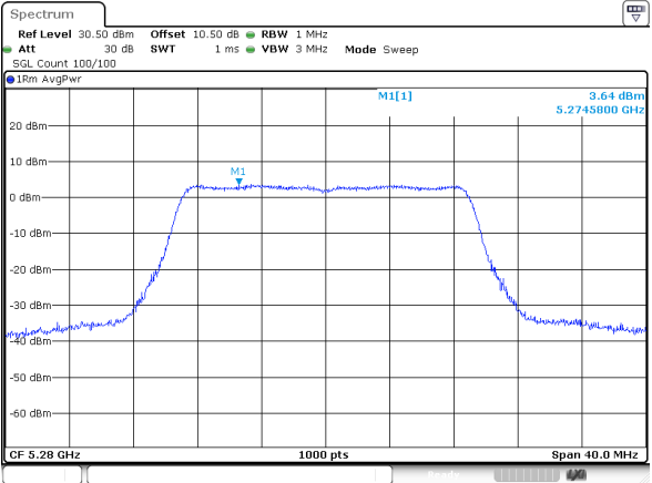
802.11ac20_5280MHz
