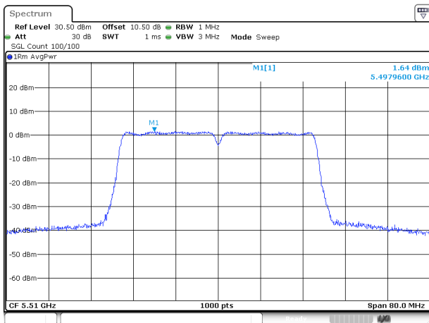
802.11ac40_5510MHz
