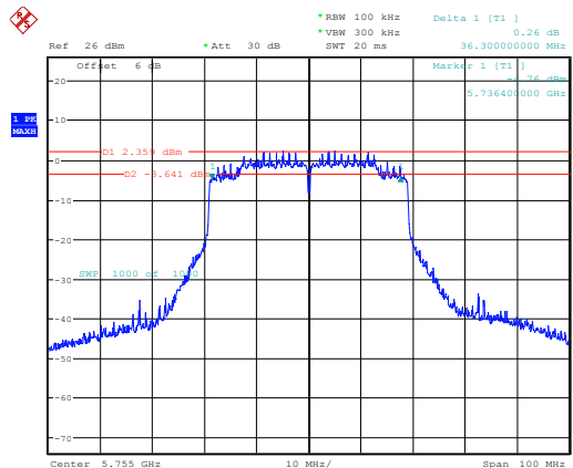
802.11ax40_5755MHz_Chain 0
