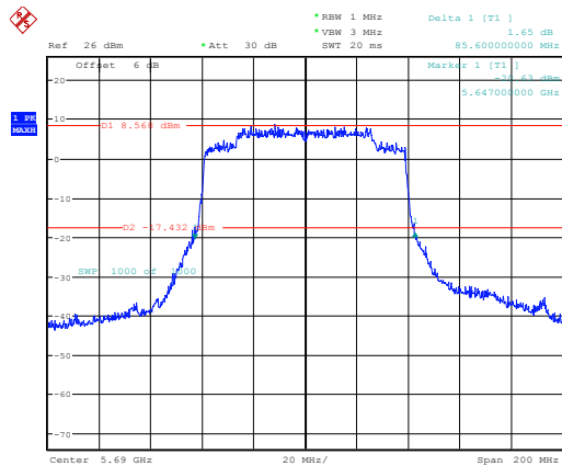
802.11ax80_5690MHz_Chain 0
