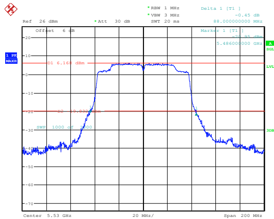
802.11ac80_5530MHz_Chain 0
