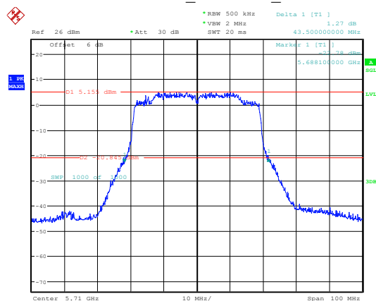
802.11ax40_5710MHz_Chain 1
