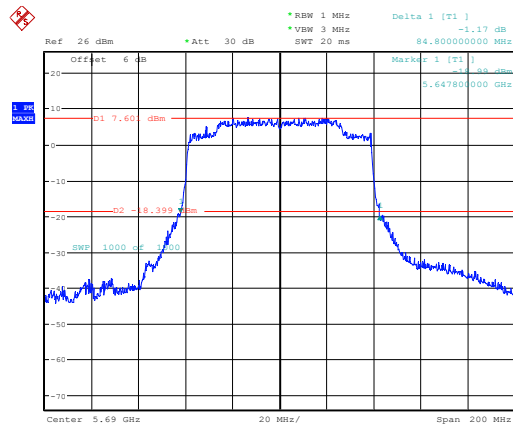
802.11ax80_5690MHz_Chain 1
