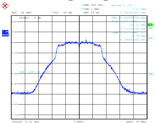
802.11a_5720MHz_Chain 1
