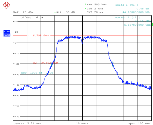
802.11ac40_5710MHz_Chain 1
