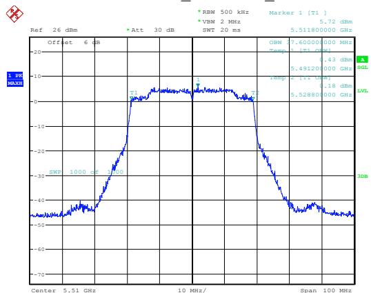
802.11ax40_5510MHz_Chain 0
