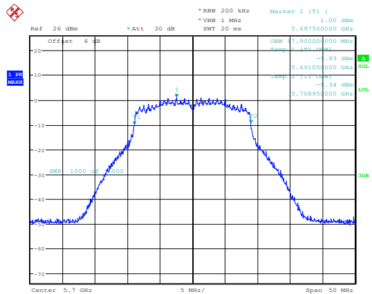
802.11ac20_5700MHz_Chain 1
