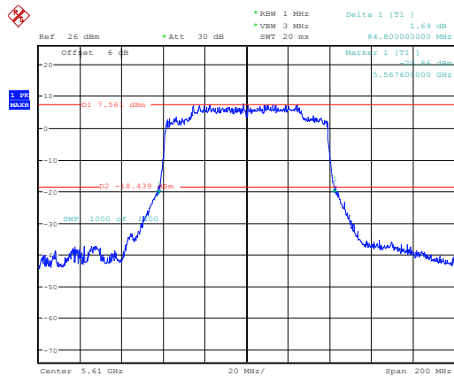
802.11ax80_5610MHz_Chain 1
