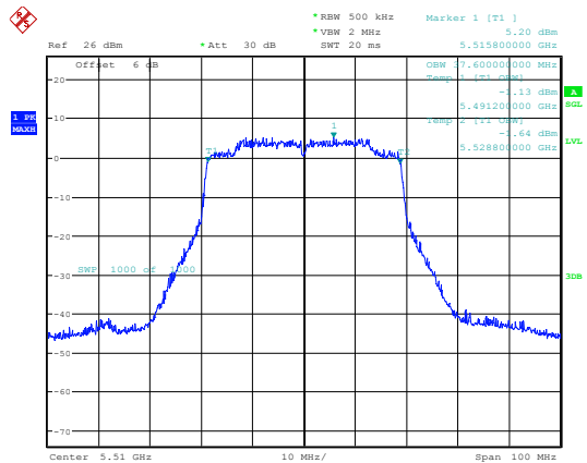
802.11ax40_5510MHz_Chain 1
