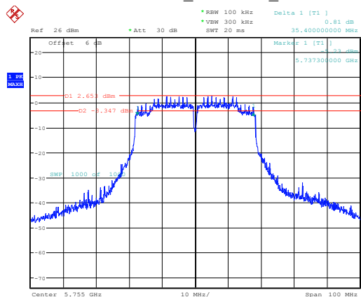
802.11ac40_5755MHz_Chain 0
