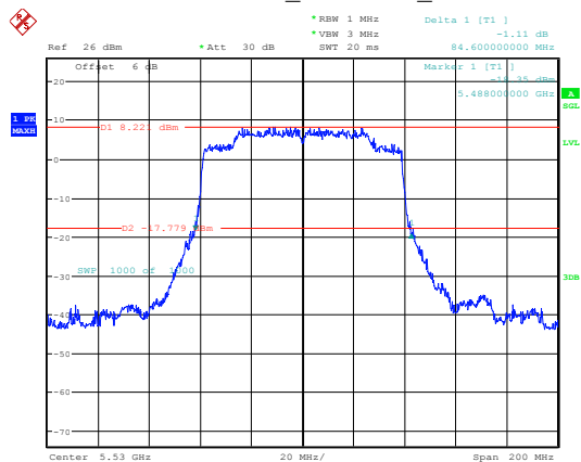
802.11ax80_5530MHz_Chain 0
