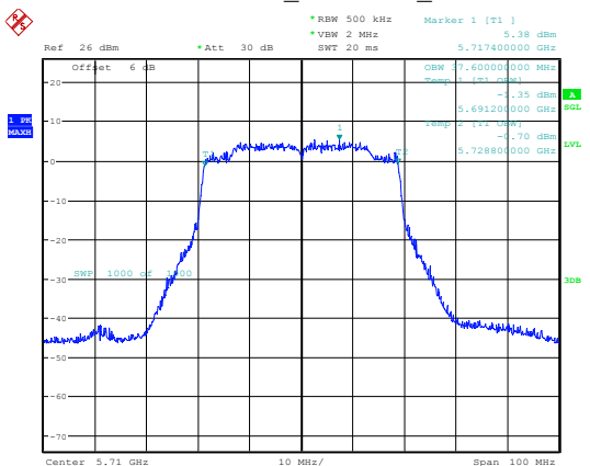
802.11ax40_5710MHz_Chain 1
