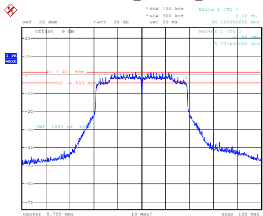
802.11ax40_5755MHz_Chain 1
