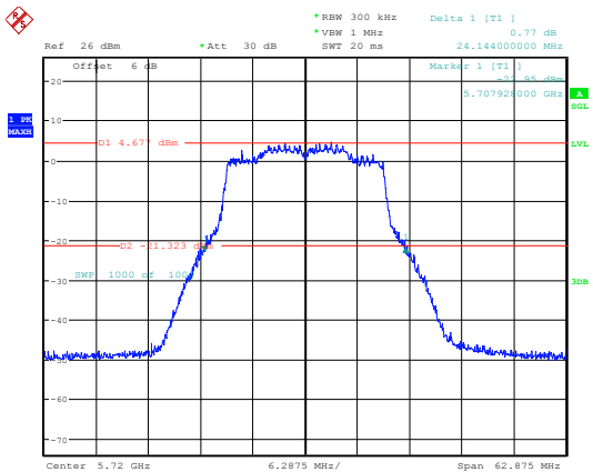
802.11ax20_5720MHz_Chain 1
