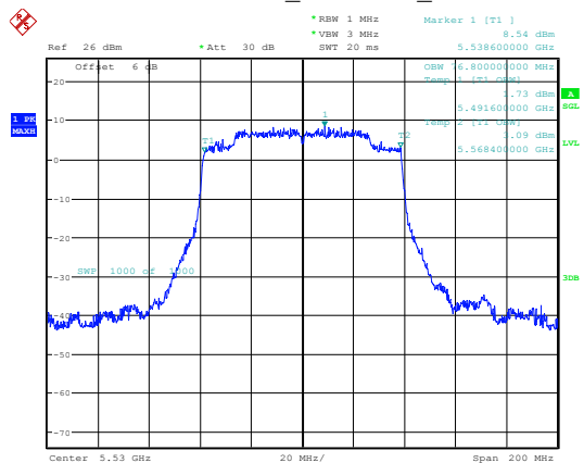
802.11ax80_5530MHz_Chain 0
