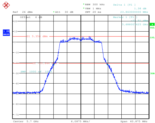
802.11ax20_5700MHz_Chain 1
