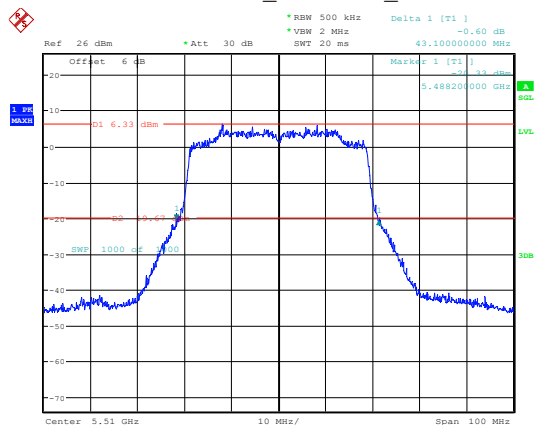
802.11ax40_5510MHz_Chain 1
