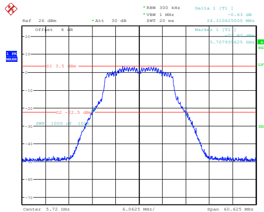
802.11ac20_5720MHz_Chain 1
