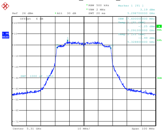
802.11ax40_5310MHz_Chain 1
