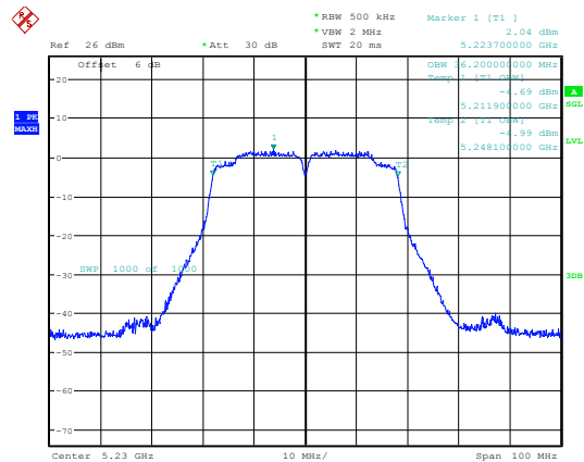
802.11ac40_5230MHz_Chain 1
