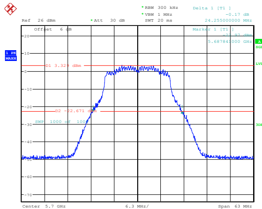
802.11ac20_5700MHz_Chain 1
