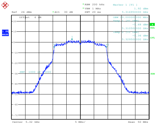
802.11ax20_5320MHz_Chain 1
