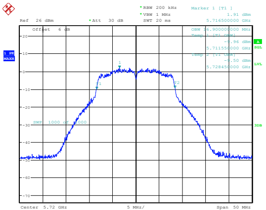
802.11a_5720MHz_Chain 0
