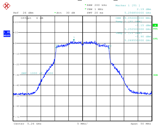
802.11ax20_5260MHz_Chain 1
