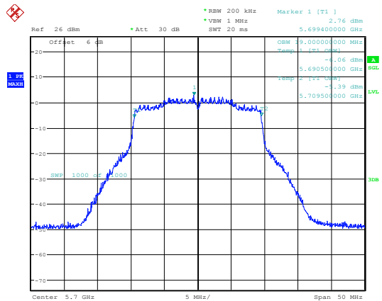
802.11ax20_5700MHz_Chain 1
