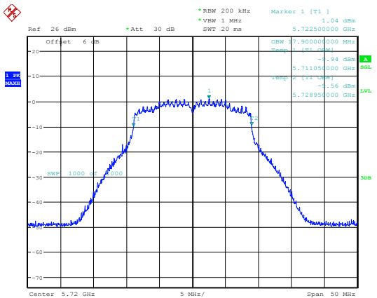
802.11ac20_5720MHz_Chain 1
