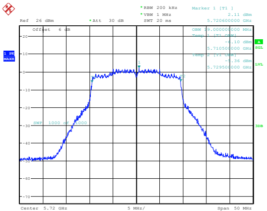
802.11ax20_5720MHz_Chain 1
