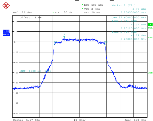
802.11ax40_5270MHz_Chain 0
