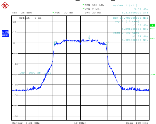
802.11ax40_5310MHz_Chain 0
