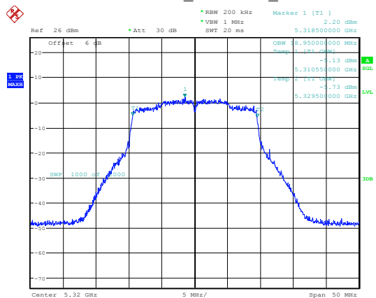
802.11ax20_5320MHz_Chain 0
