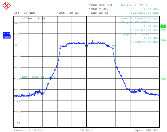
802.11ac40_5190MHz_Chain 0
