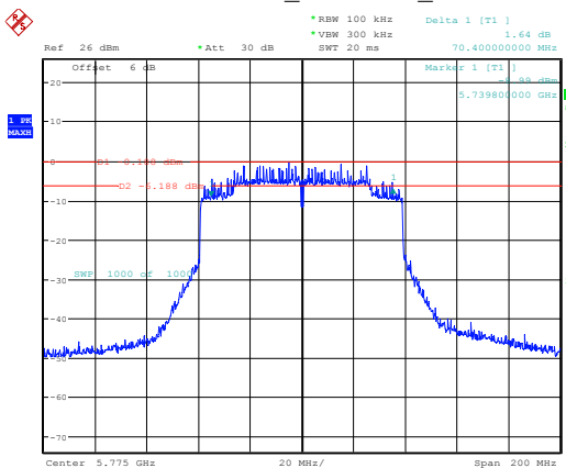
802.11ax80_5775MHz_Chain 1
