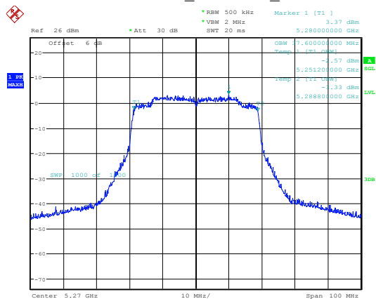
802.11ax40_5270MHz_Chain 1
