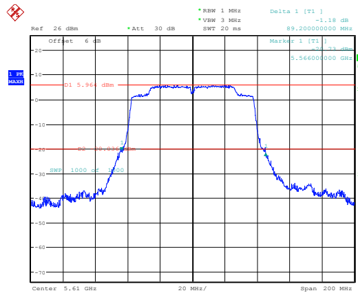
802.11ac80_5610MHz_Chain 0
