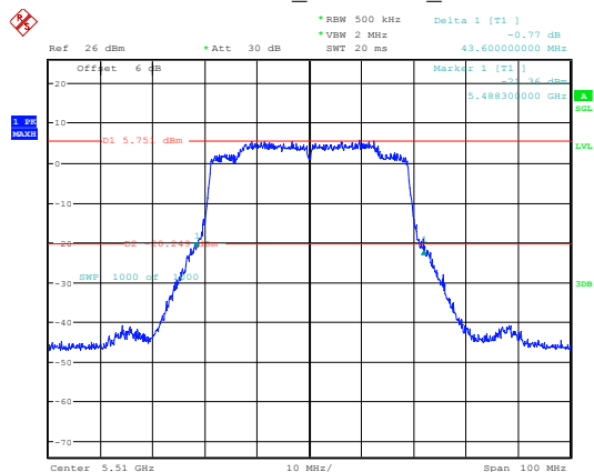
802.11ax40_5510MHz_Chain 0
