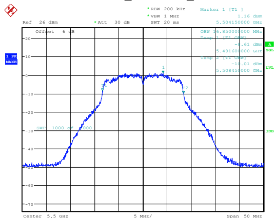
802.11a_5500MHz_Chain 1
