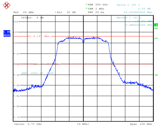
802.11ac40_5710MHz_Chain 0
