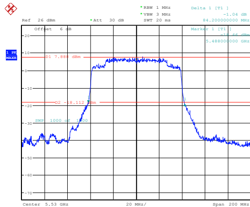
802.11ax80_5530MHz_Chain 1
