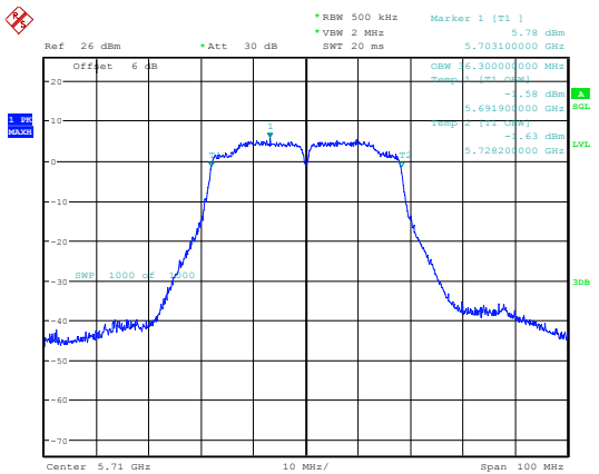
802.11ac40_5710MHz_Chain 0
