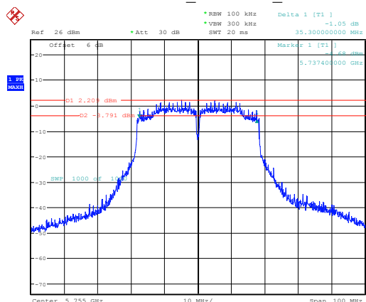
802.11ac40_5755MHz_Chain 1
