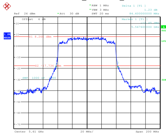
802.11ax80_5610MHz_Chain 0
