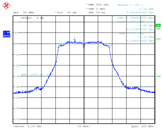
802.11ac40_5190MHz_Chain 1
