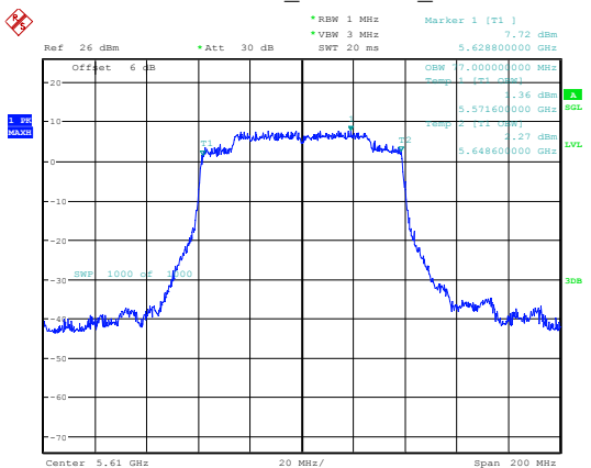
802.11ax80_5610MHz_Chain 0
