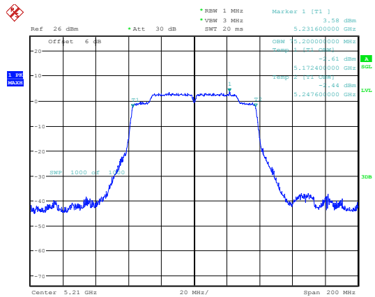
802.11ac80_5210MHz_Chain 0
