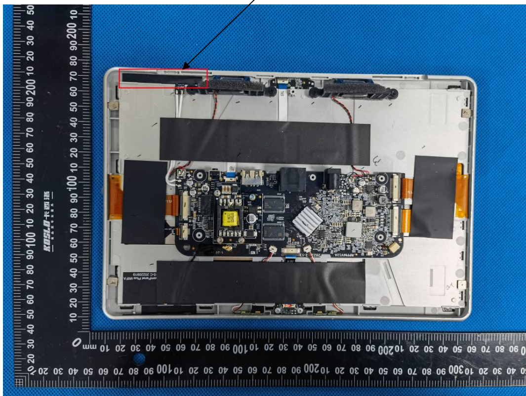
NFC ANT
