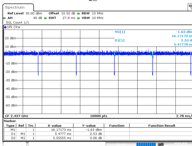
802.11g_2437MHz
