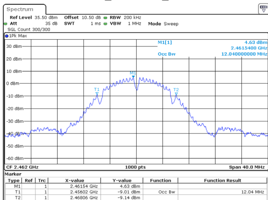
802.11b_2462MHz_Chain 1
