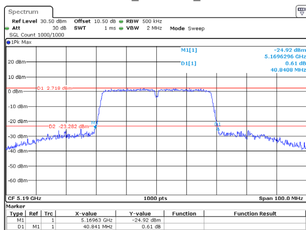
802.11ac40_5190MHz_Chain 1
