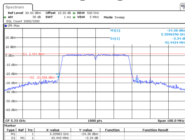
802.11ac40_5230MHz_Chain 1
