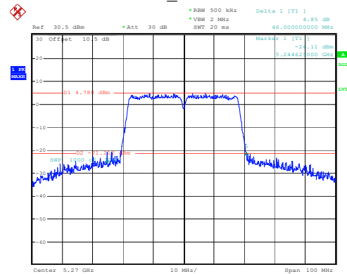
802.11n40_5270MHz 46MHz
