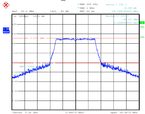
802.11n20_5320MHz 24.749MHz
