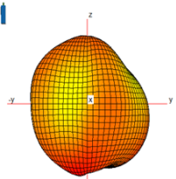
3D天线图
