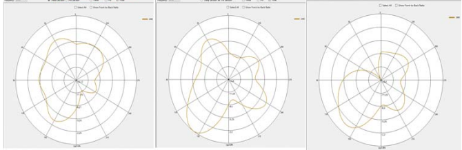
2D天线图 (X-Y,X-Z,Y-Z)
