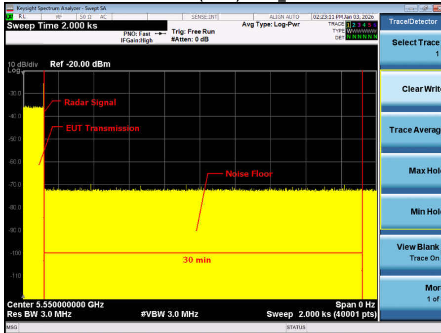
IEEE 802.11ax(HE40) Mode_5550MHz
