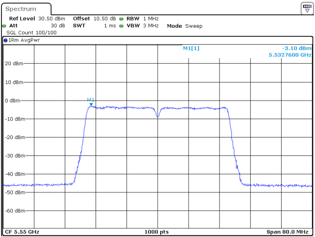
802.11ac40_5550MHz
