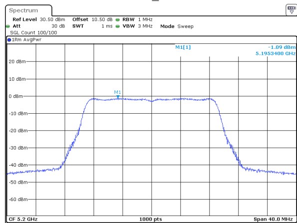
802.11ac20_5200MHz
