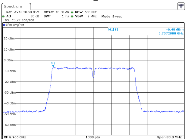
802.11ac40_5755MHz
