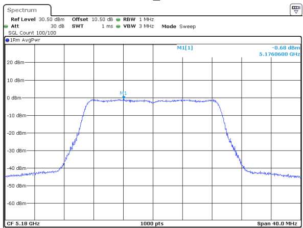
802.11ac20_5180MHz
