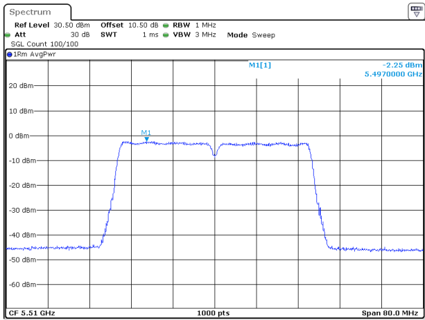
802.11ac40_5510MHz
