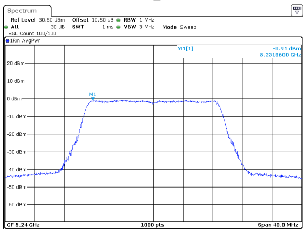
802.11ac20_5240MHz
