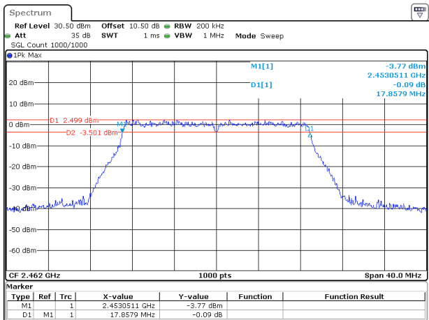
802.11n20_2462MHz
