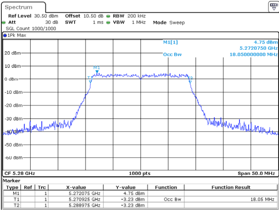
802.11ac20_5280MHz
