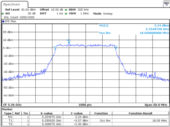
802.11ac20_5260MHz
