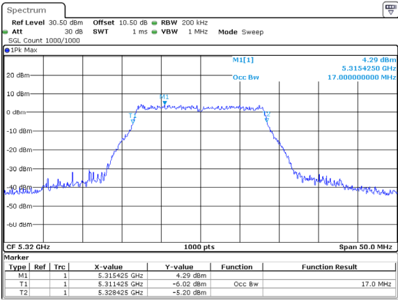
802.11a_5320MHz
