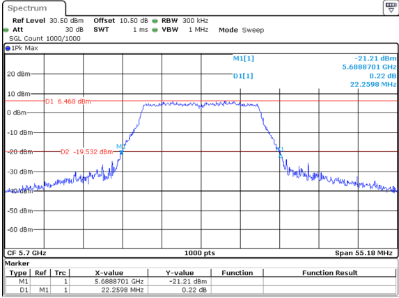
802.11a_5700MHz
