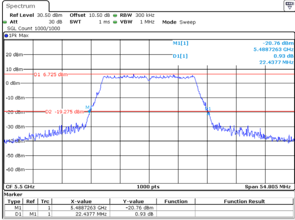
802.11ac20_5500MHz
