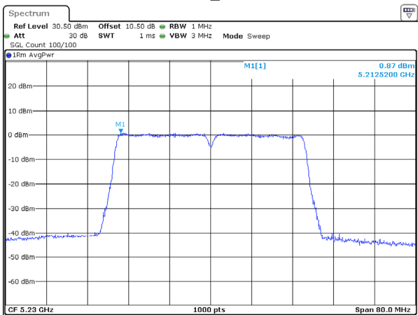
802.11ac40_5230MHz
