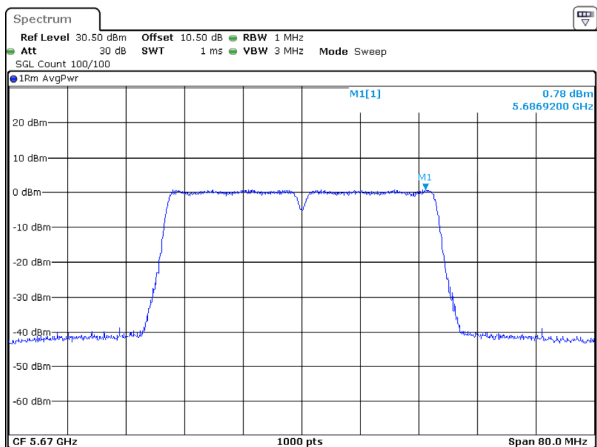
802.11ac40_5670MHz
