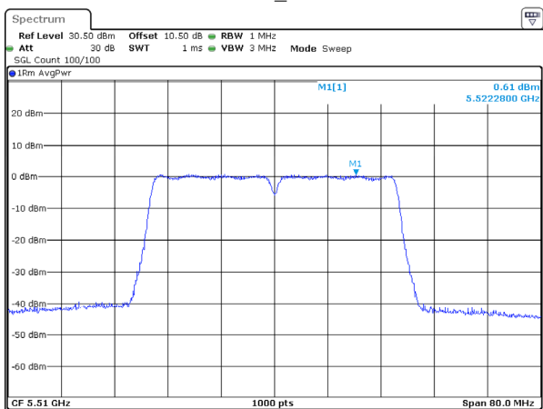
802.11ac40_5510MHz
