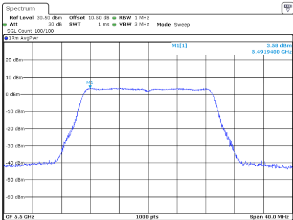
802.11ac20_5500MHz
