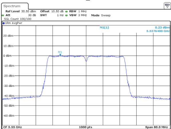
802.11ac40_5550MHz
