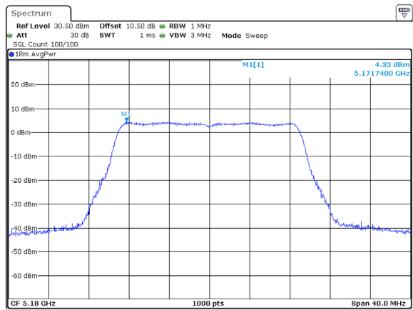
802.11ac20_5180MHz
