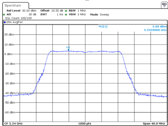
802.11ac20_5240MHz
