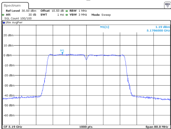
802.11ac40_5190MHz
