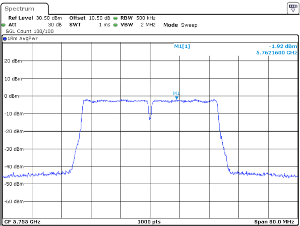
802.11ac40_5755MHz
