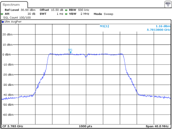
802.11ac20_5785MHz
