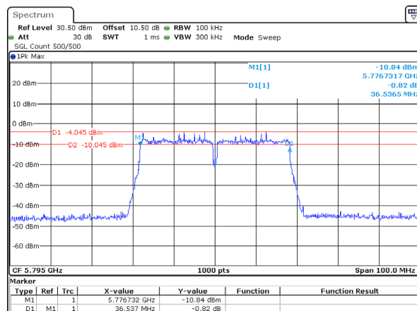
802.11ac40_5795MHz
