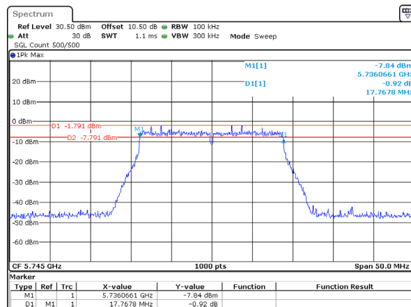
802.11ac20_5745MHz
