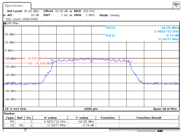
802.11n20_2412MHz_Chain 1
