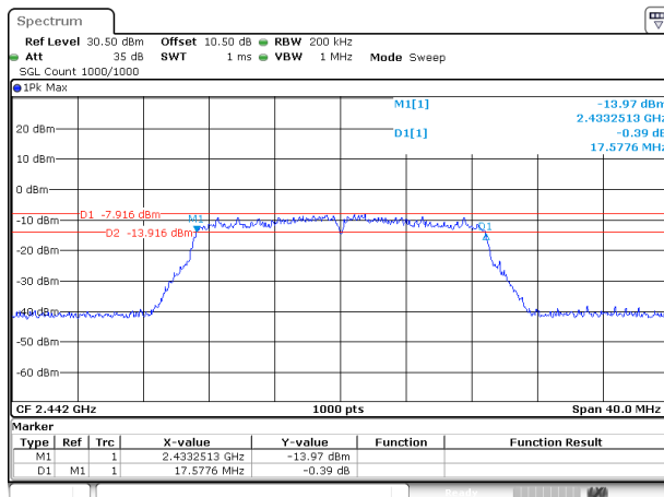
802.11n20_2442MHz_Chain 1
