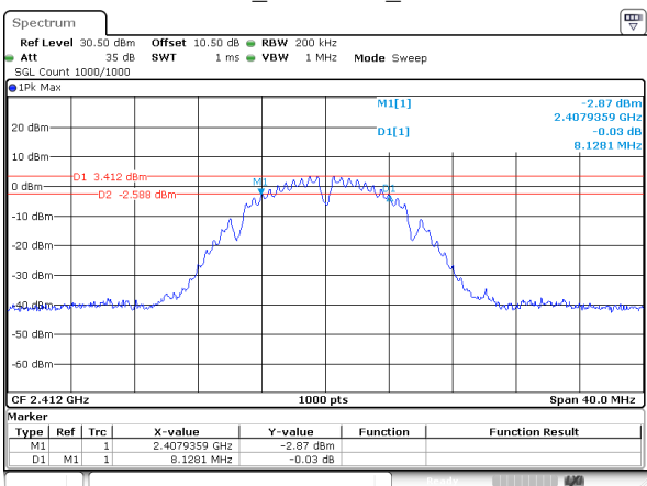
802.11b_2412MHz_Chain 1
