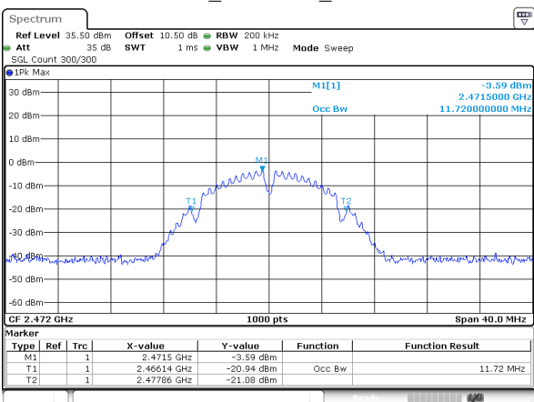
802.11b_2472MHz_Chain 0
