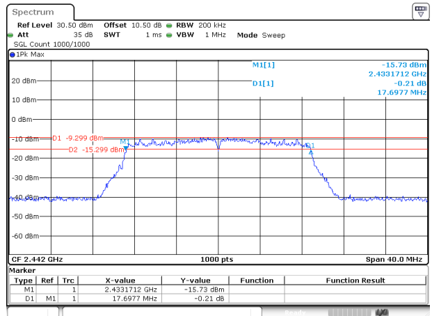
802.11n20_2442MHz_Chain 0
