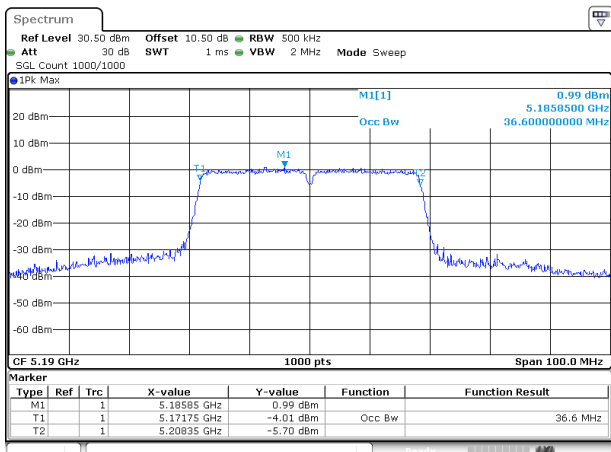
802.11ac40_5190MHz_Chain 0
