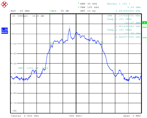
2DH1_Low 1.148MHz
