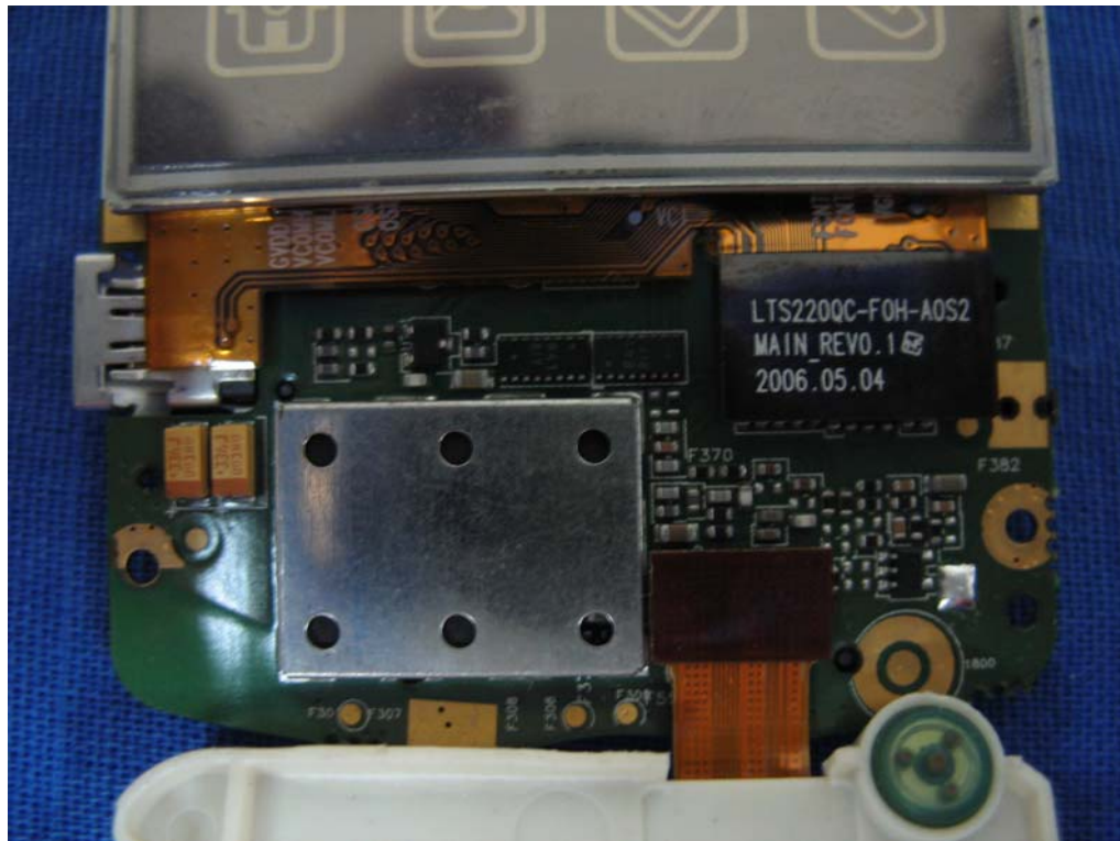
(17) EUT Photo
