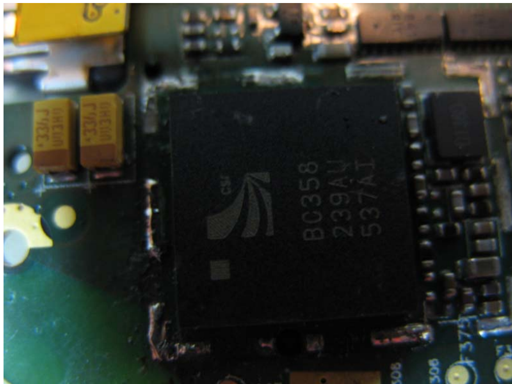
(18) EUT Photo
