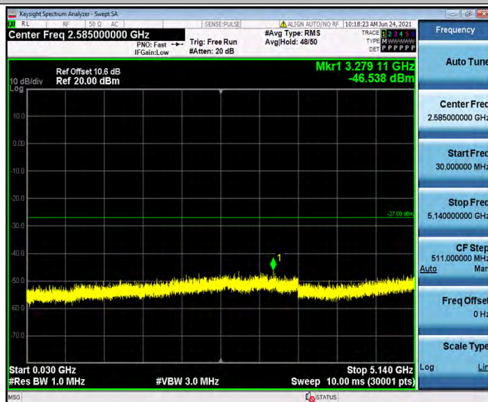
11N20_Ant2_5200_30~5140
