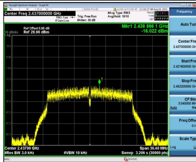
11G_Ant2_2437
