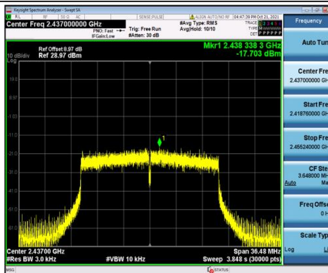
11AX20MIMO_Ant1_2437
