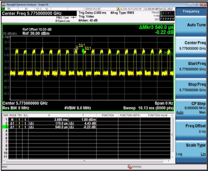
11AX80MIMO_Ant2_5775
