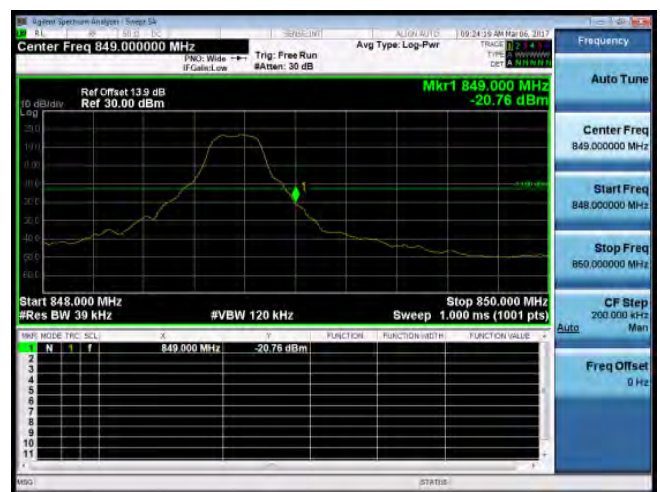
Band Edge_Band5_3MHz_QPSK_1_14_HighCH20635-847.5
