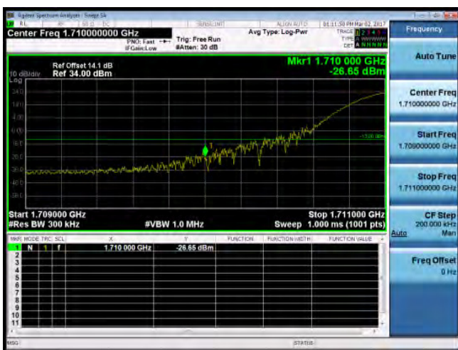
Band Edge_Band4_20MHz_QPSK_1_0_LowCH20050-1720
