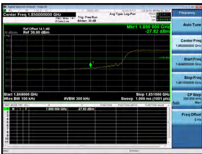
Band Edge_Band2_10MHz_QPSK_50_0_LowCH18650-1855
