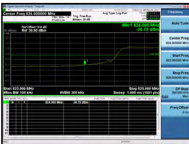
Band Edge_Band5_10MHz_QPSK_50_0_LowCH20450-829
