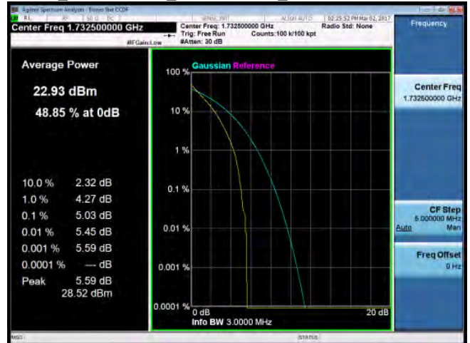
LTE_Band4 3MHz_16-QAM 15 0_MidCH20175-1732.5
