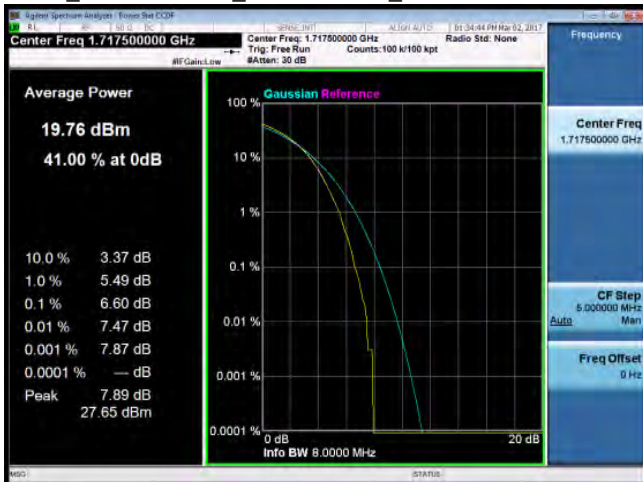
LTE_Band4 15MHz_16-QAM 75 0_LowCH20025-1717.5
