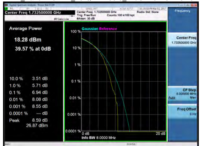
LTE_Band4 20MHz_16-QAM 100 0_MidCH20175-1732.5
