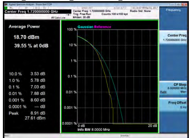
LTE_Band4 20MHz_16-QAM 100 0_LowCH20050-1720
