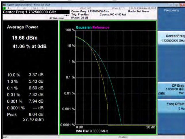
LTE_Band4 15MHz_16-QAM 75 0_MidCH20175-1732.5
