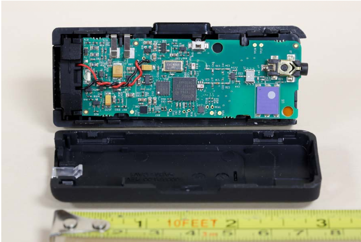
Internal Photos – T5V01EXECCMICWR and 6455A-01EXECCMICWR
