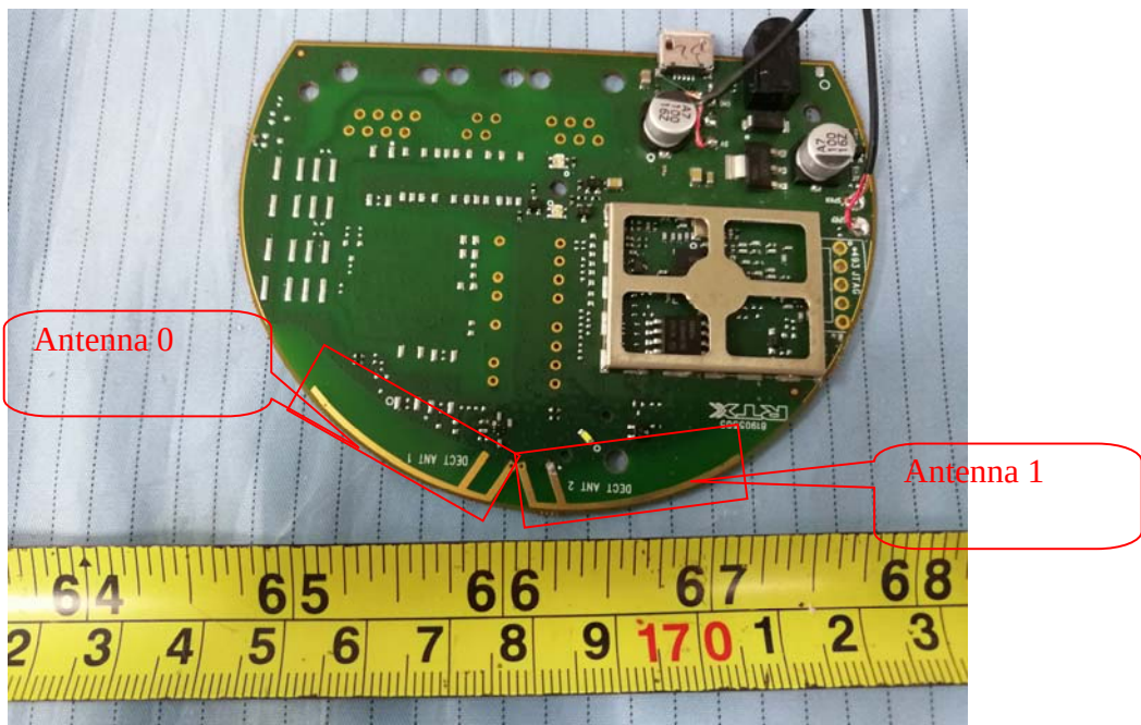
EUT – Mian Board Top View
