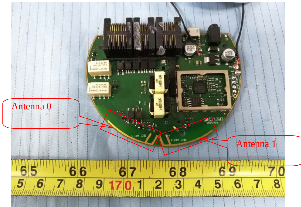
EUT – Mian Board Top View
