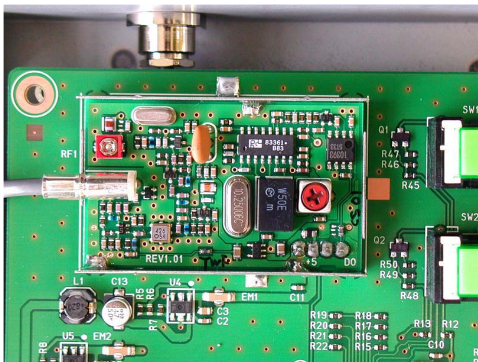
RX module (Top)
