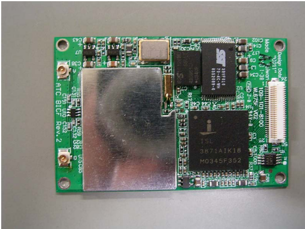
WLAN Module (Component Side)
