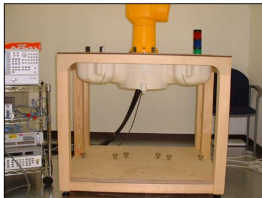
SAM Twin Phantom
