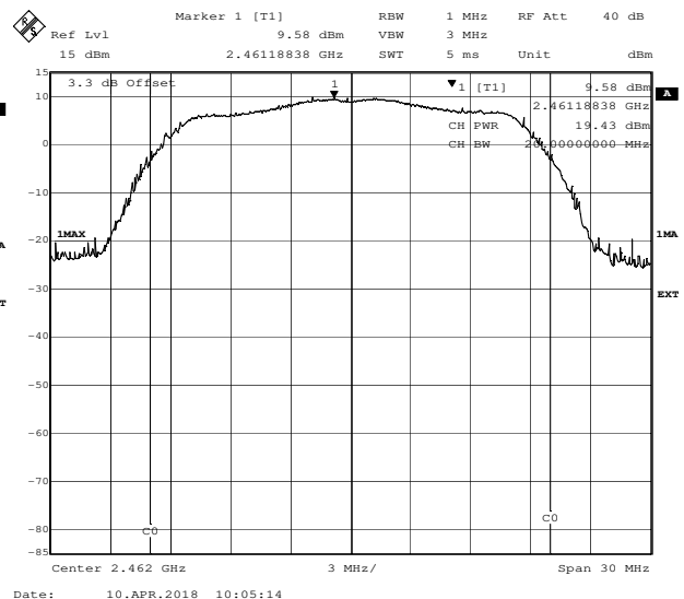
Mode n MIMO, Ant 2
