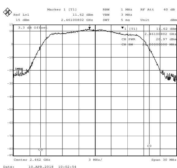
Mode n MIMO, Ant 1
