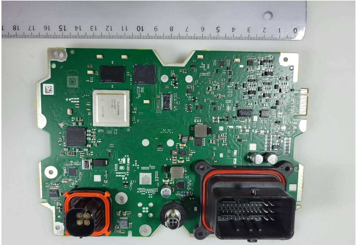
PCBA Z068 4010 bottom
