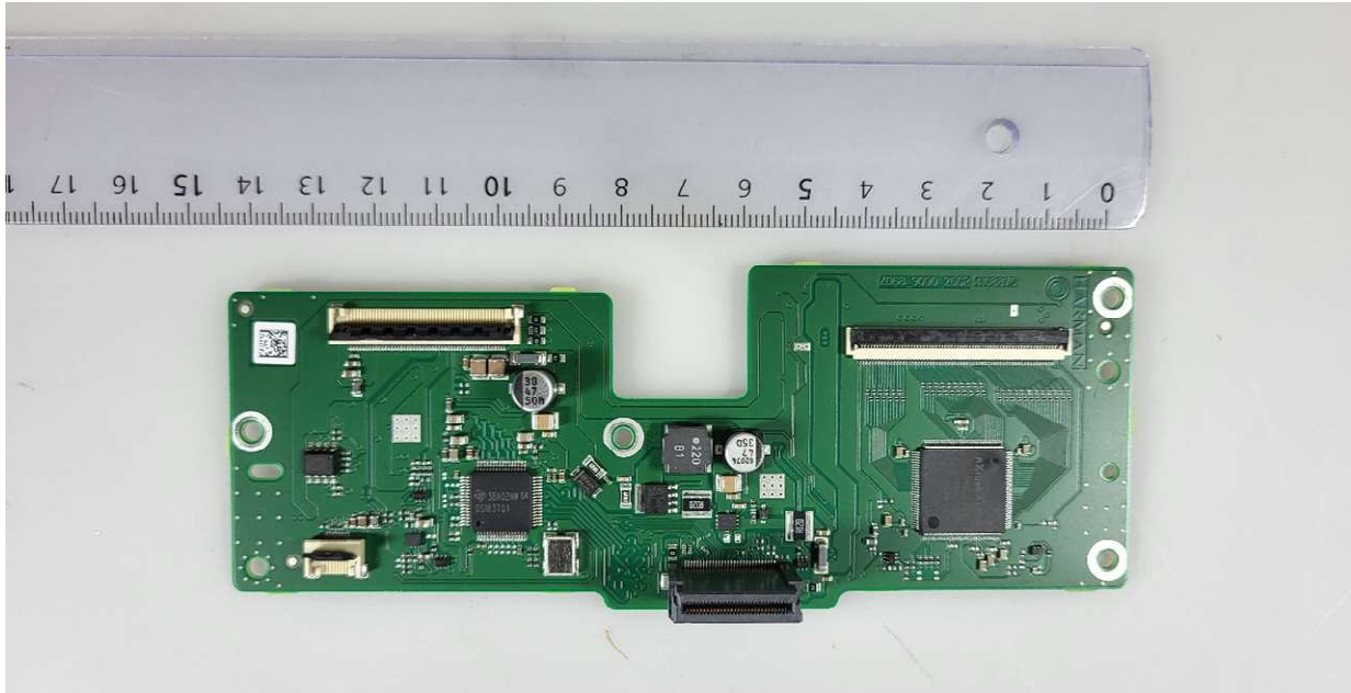
PCBA Z068 9090 bottom
