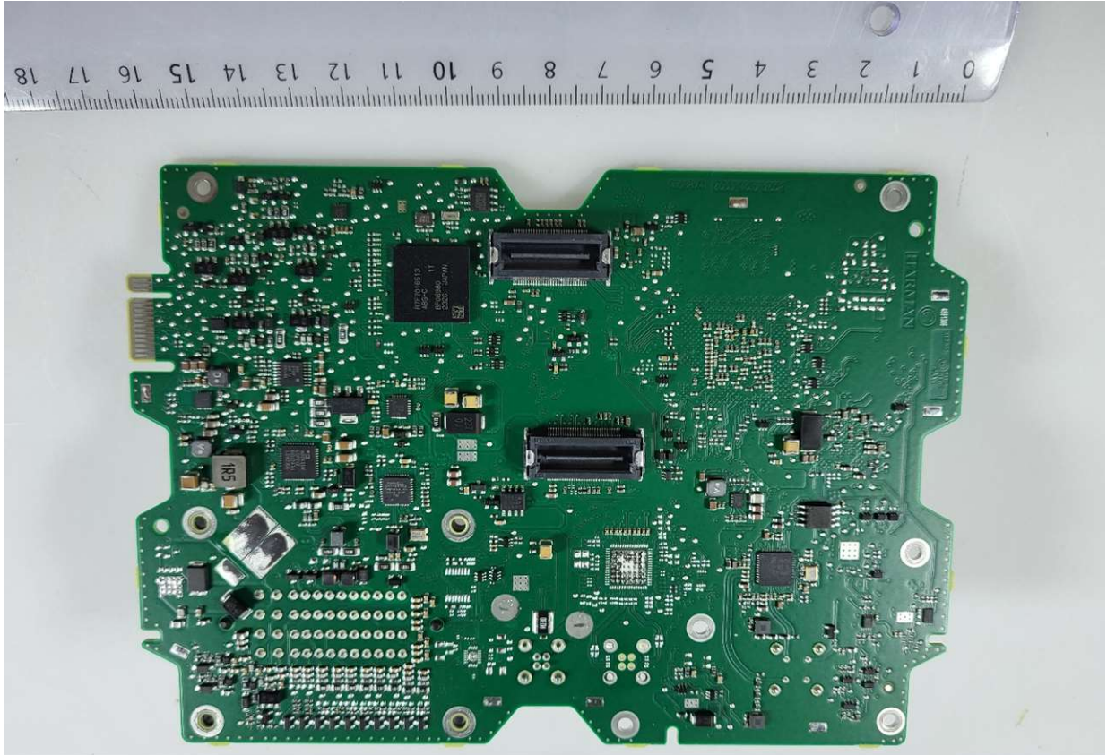
PCBA Z068 4010 bottom
