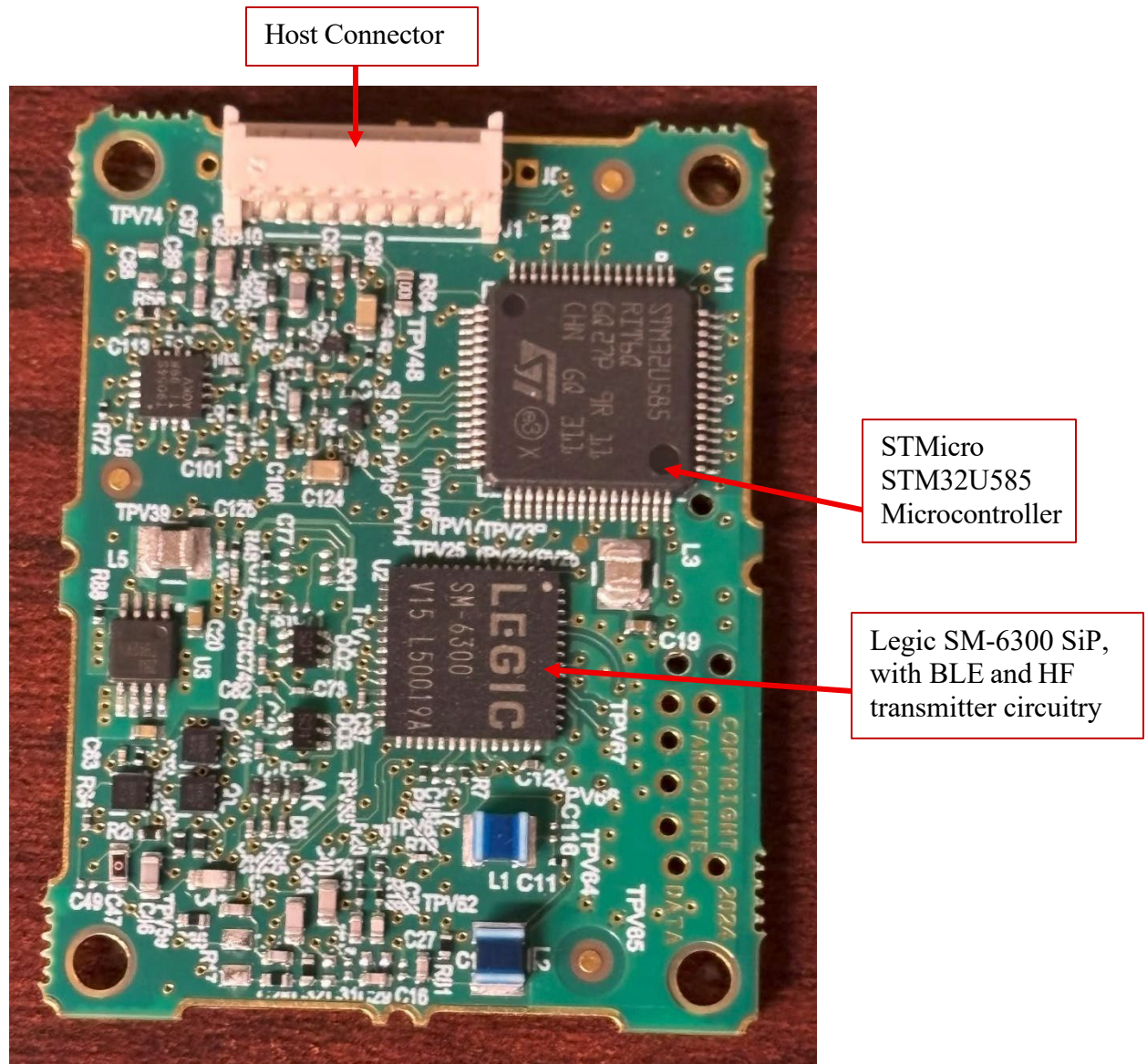
CSM-200 Module – Top
