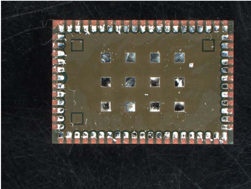
Bluetooth Module
