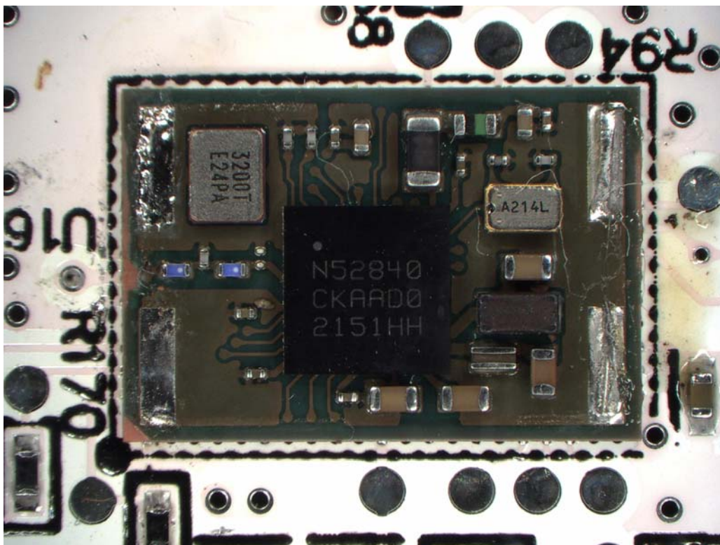
Bluetooth Module
