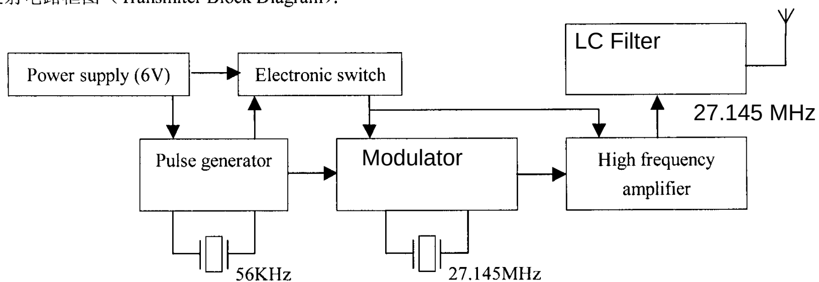
发射电路框图 (Transmitter Block Diagram):
