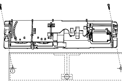
Montage mit Bohrschablone
