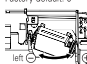
Radar module
