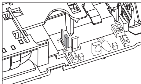
Cavalier pour définir le type de sortie AIR
