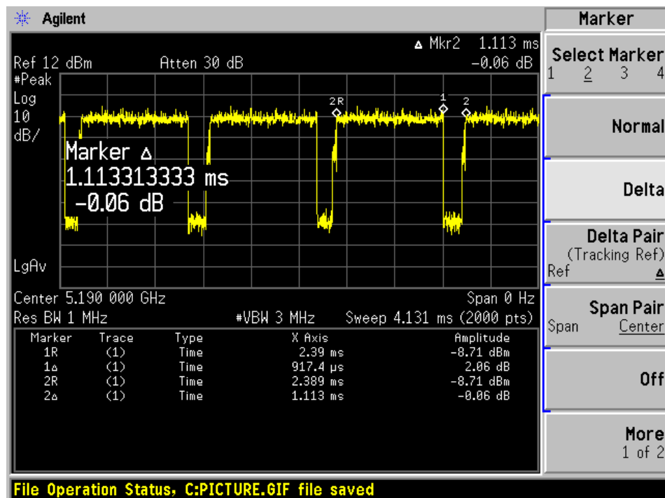
802.11n/ac40 mode
