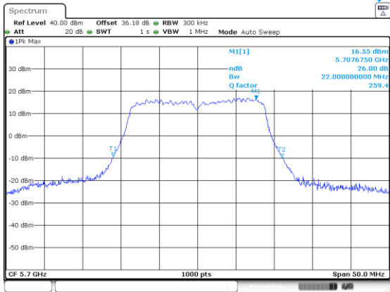
n/ac20_5700_Ant B
