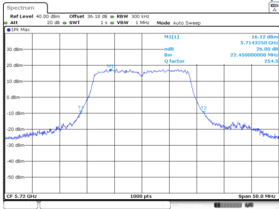
n/ac20_5720_Ant B
