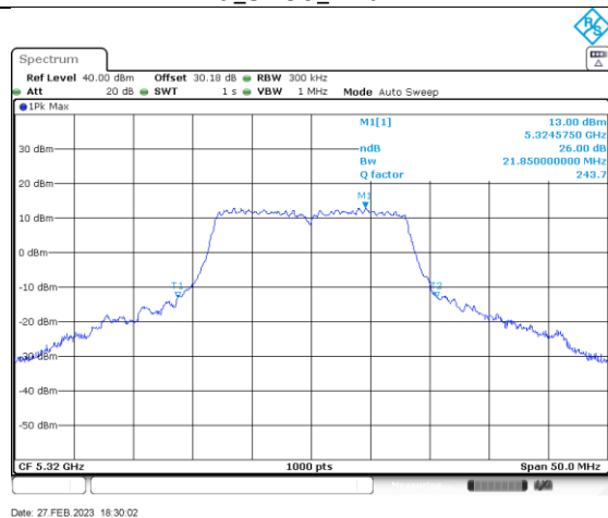
a_5320_Ant A
