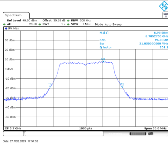
a_5700_Ant B
