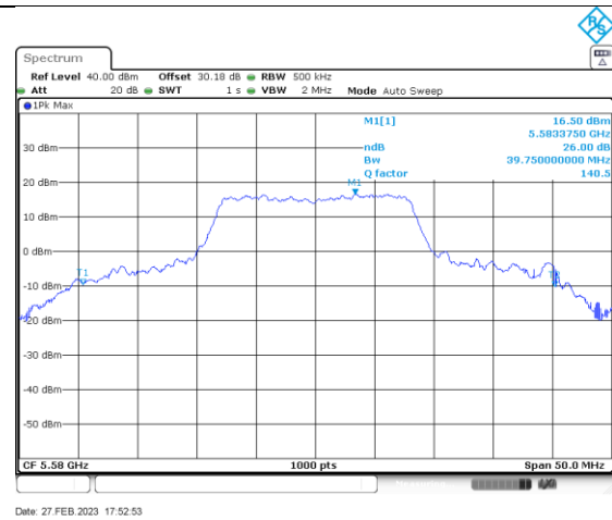
a_5580_Ant B
