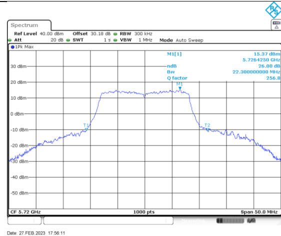
a_5720_Ant B
