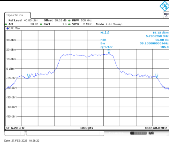
a_5280_Ant A
