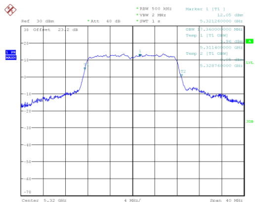
a_5320_Ant B
