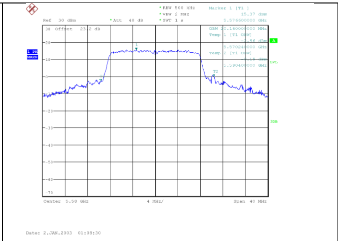
a_5580_Ant B
