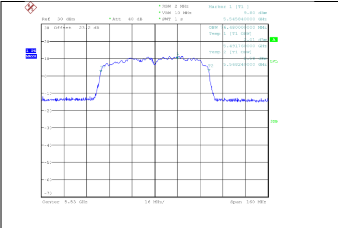
ac80_5530_Ant A
