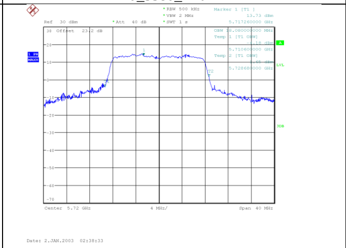
a_5720_Ant B
