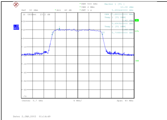
n/ac20_5700_Ant B
