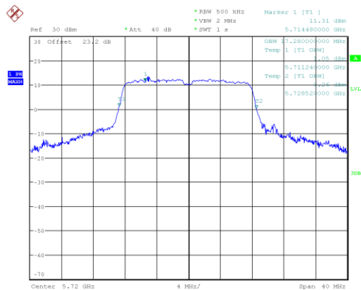
a_5720_Ant A
