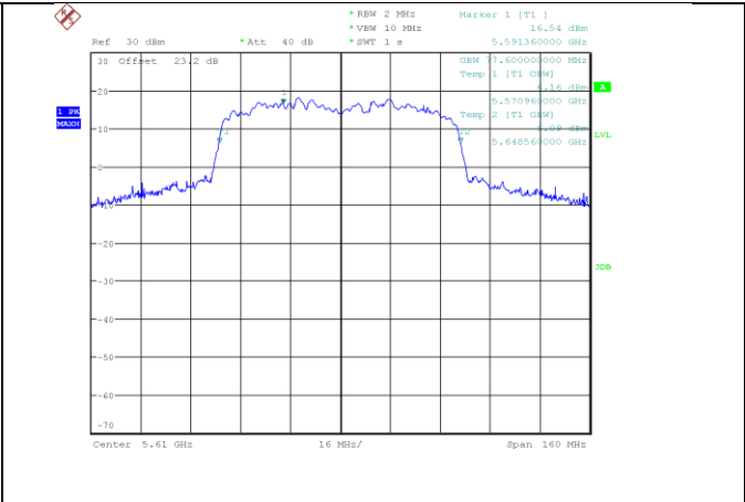
ac80_5610_Ant A
