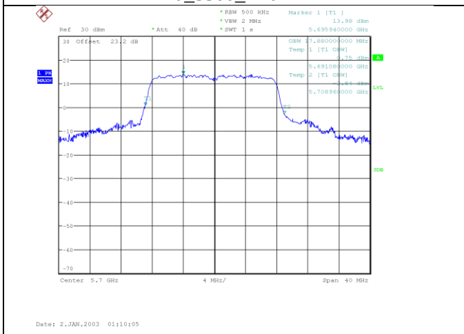
a_5700_Ant B
