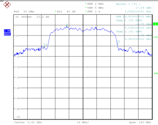
ac80_5610_Ant B
