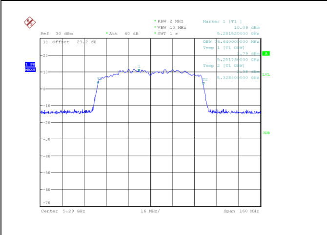
ac80-5290_Ant B
