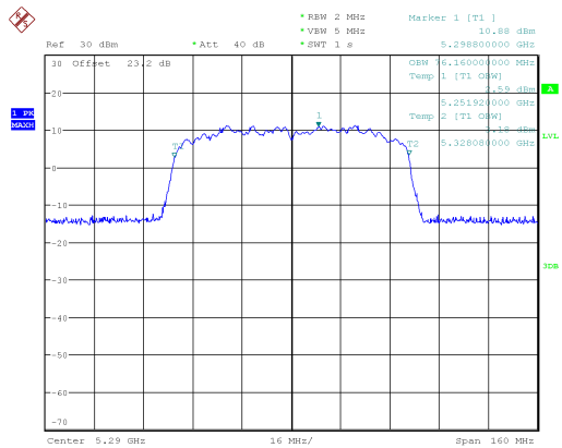
ac80_5290_Ant A
