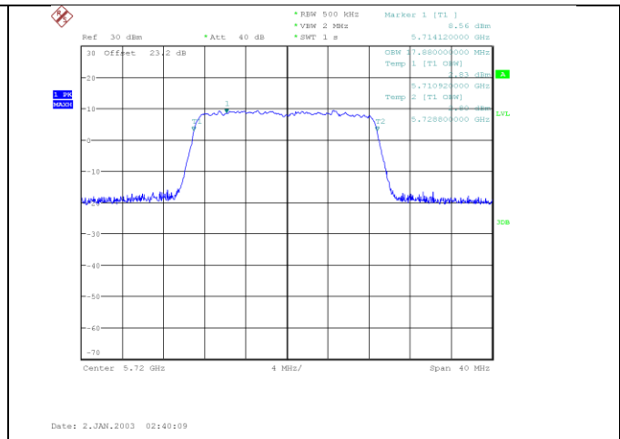
n/ac20_5720_Ant B
