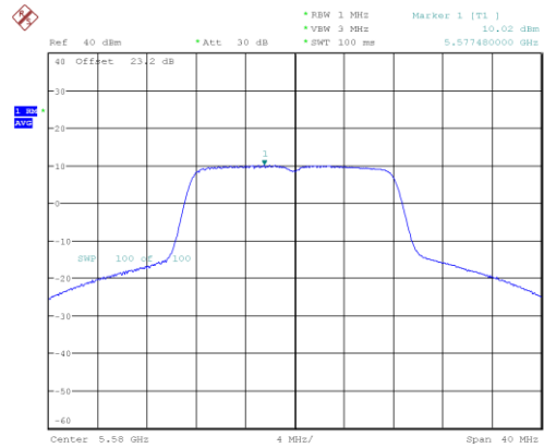
a_5580_Ant A
