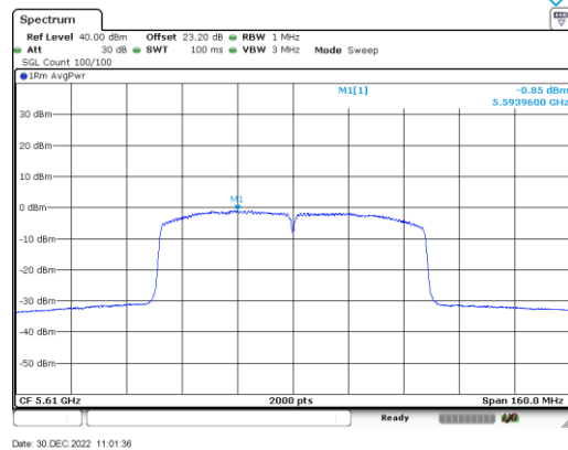
ac80_5610_Ant A
