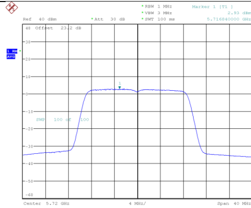
n/ac20_5720_Ant A
