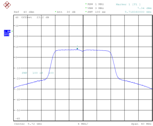
a_5720_Ant A
