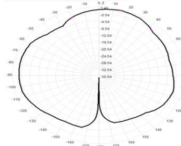
5150.0MHz Total(E1-XZ), Max= 2.67dBi
