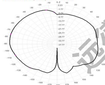
5850.0MHz Total(E1-XZ), Max= 0.64dBi
