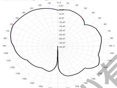
5450.0MHz Total(E2-YZ), Max= 3.53dBi
