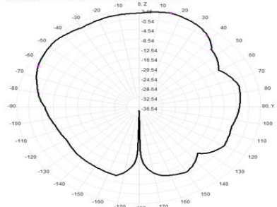
5150.0MHz Total(E2-YZ), Max= 3.46dBi
