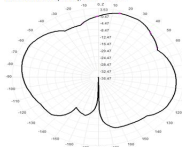
5450.0MHz Total(E1-XZ), Max= 1.96dBi
