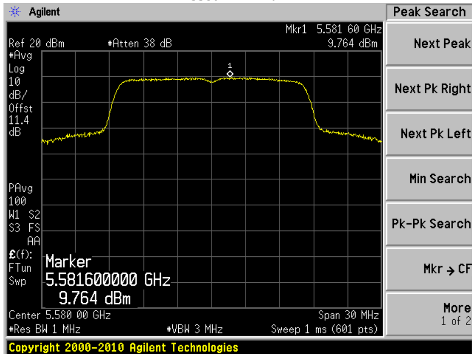
5580MHz Ant B
